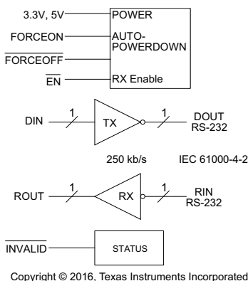
ブロック図
