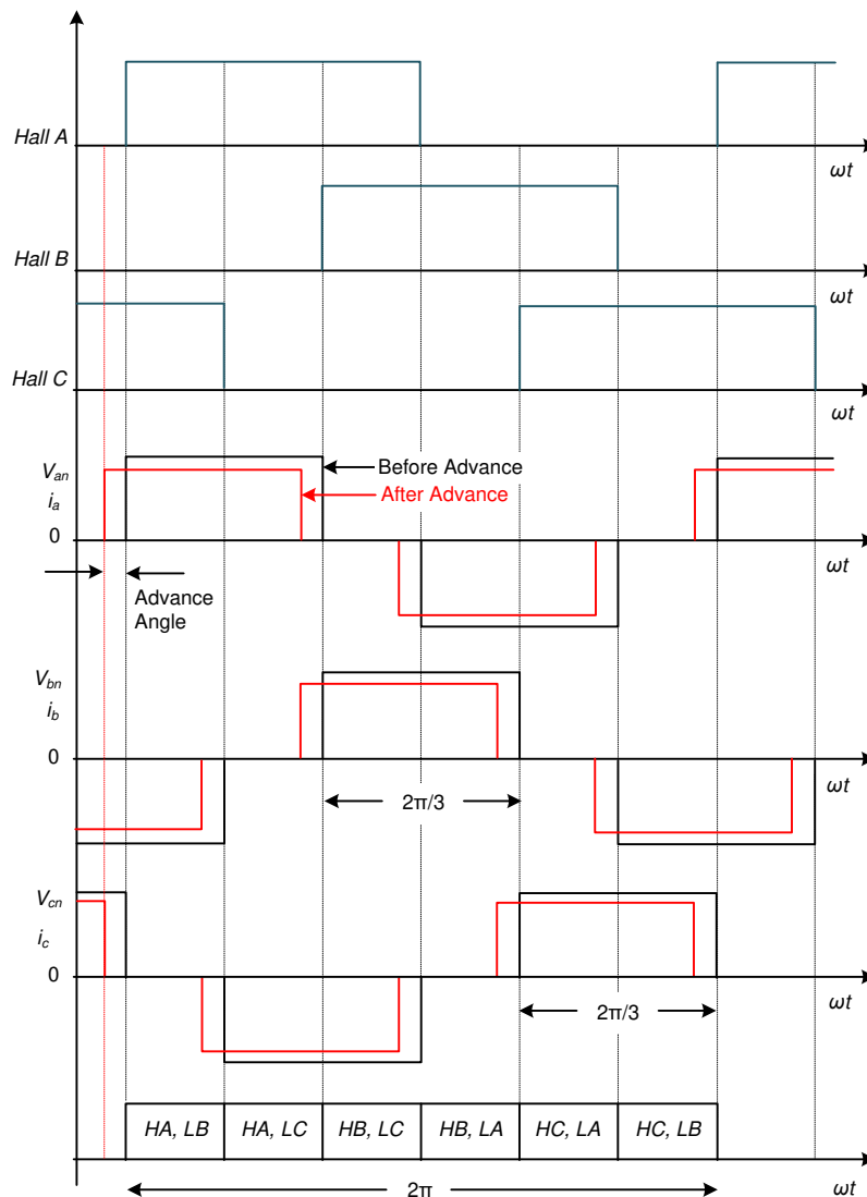
図 7-28. Advance Angle
