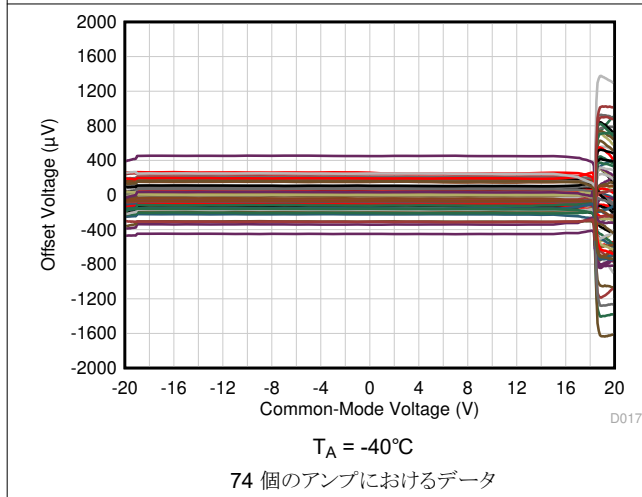
図 5-9. オフセット電圧と同相電圧との関係
