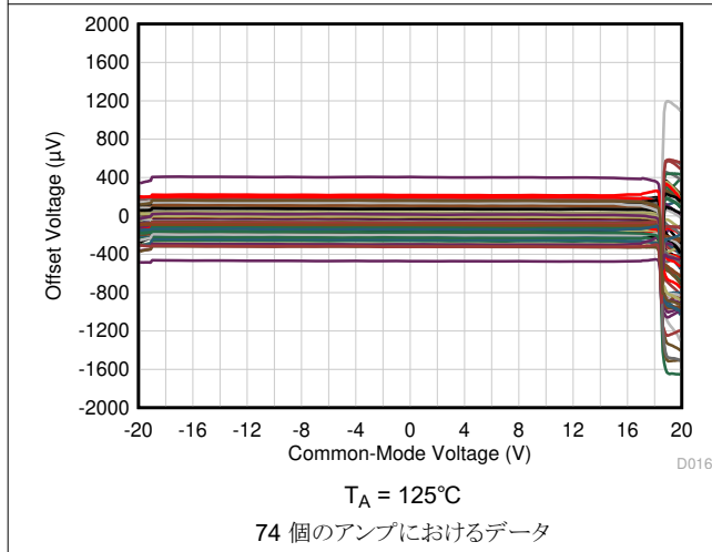
図 5-7. オフセット電圧と同相電圧との関係
