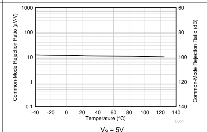
図 5-22. CMRR と温度との関係
