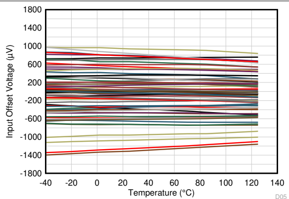
図 5-8. 入力オフセット電圧と温度との関係
