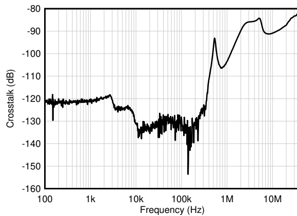
図 5-53. チャンネル セパレーション
