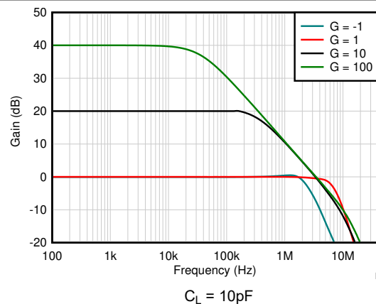
図 5-20. 閉ループゲインと周波数との関係
