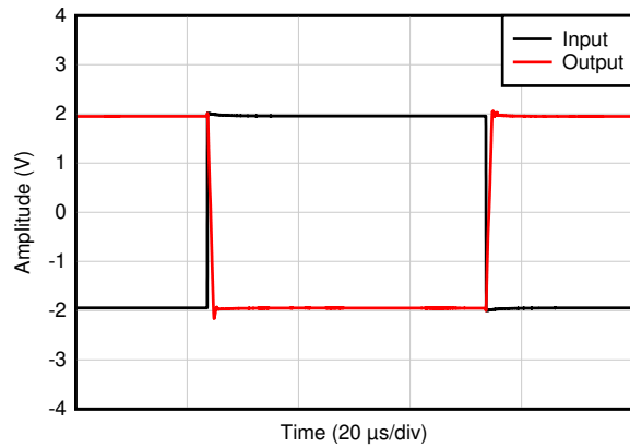
図 5-49. 大信号ステップ応答
