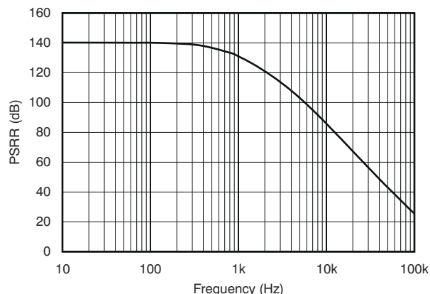
図 6-5. 電源除去比と周波数との関係
