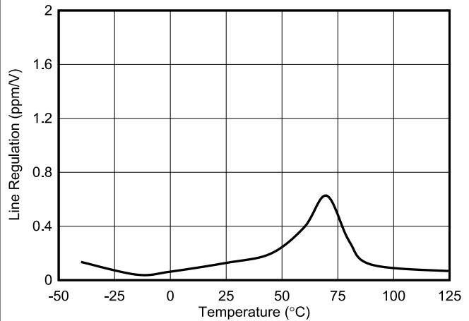
図 6-34. ラインレギュレーションと温度との関係
