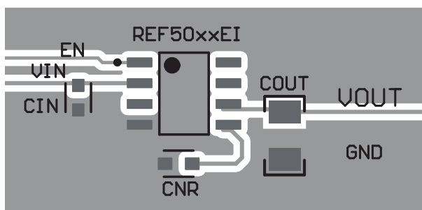
図 9-4. REF50xxEI のレイアウト例
