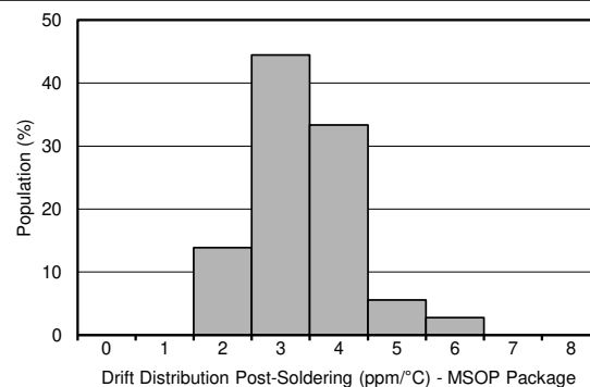
図 7-8. 半田付け後のドリフトの分散, VSSOP パッケージ
