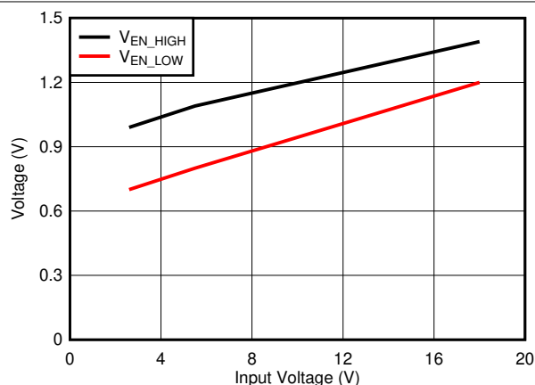
図 6-43. イネーブル スレッシュホールドと V_{IN} との関係
