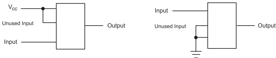
図 9-3. Layout Diagram
