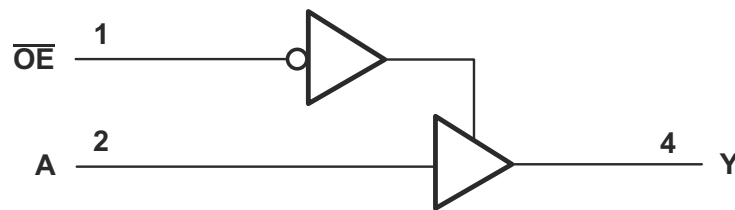
図 8-1. Logic Diagram
