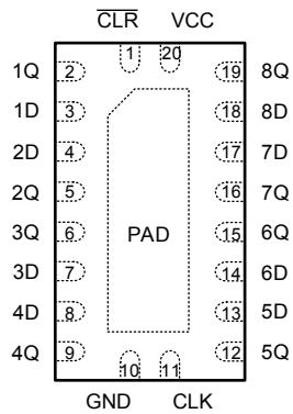
図 4-1. SN74LV8T273-Q1 RKS または RGY パッケージ (上面図)
