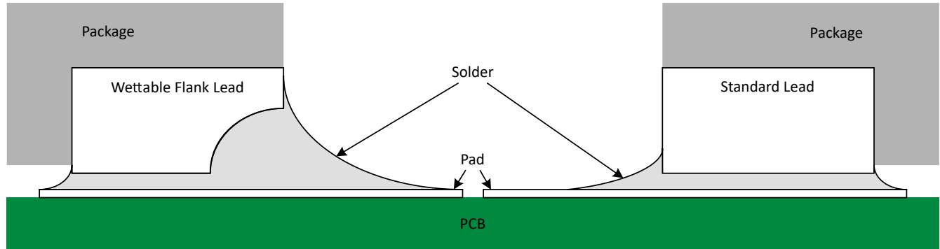
図 7-3. 半田付け後のウェットブル フランク QFN パッケージと標準 QFN パッケージの概略断面図
