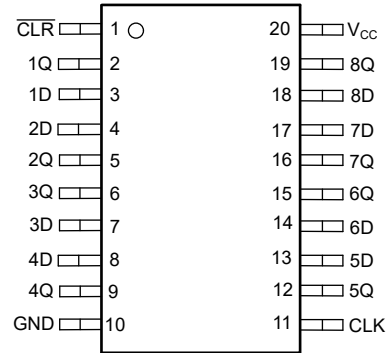
図 4-2. SN74LV8T273-Q1 PW、DGS パッケージ (上面図)
