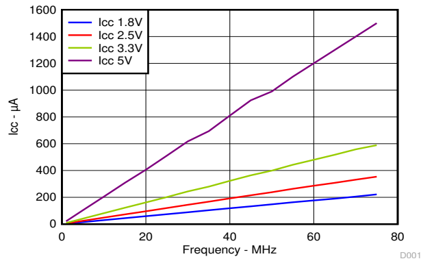
図 8-1. Icc と周波数との関係
