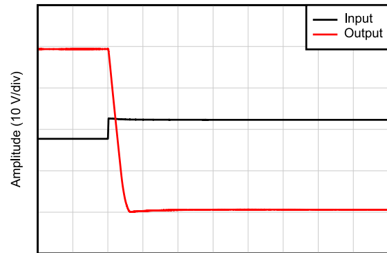
図 5-26. 位相反転が発生しない
