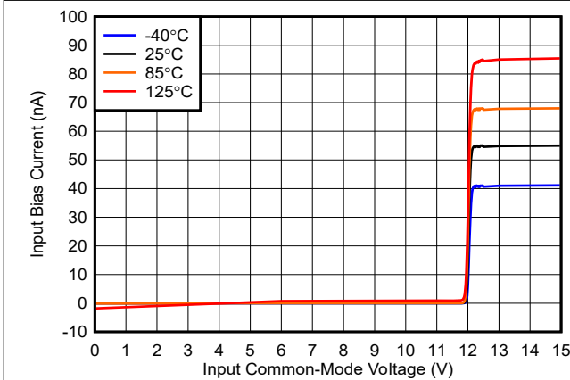
図 6-5. バイアス電流と同相との関係、12V
