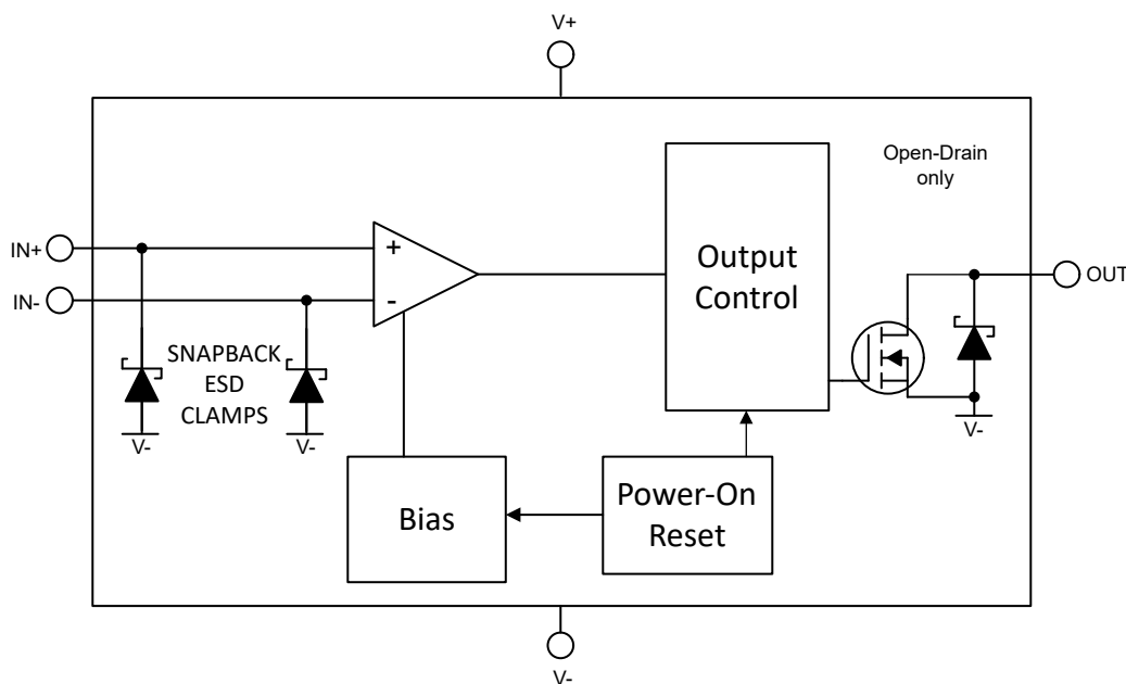
図 7-1. ブロック図
