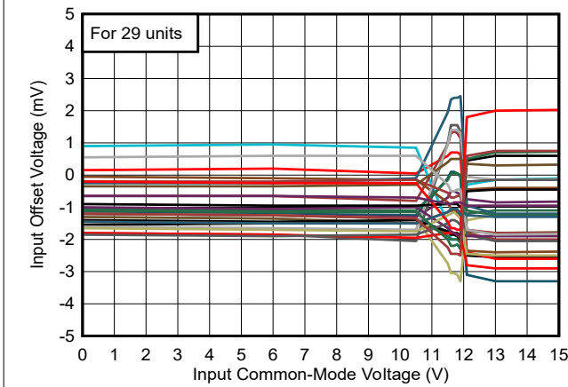
図 6-3. オフセットと同相との関係、12V
