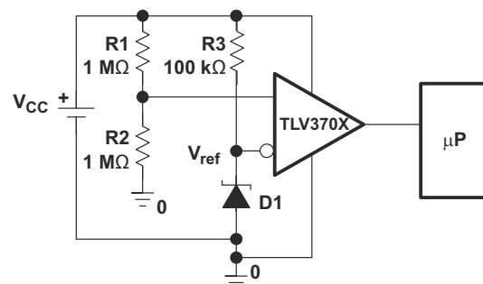
ハイサイド電圧検出回路
