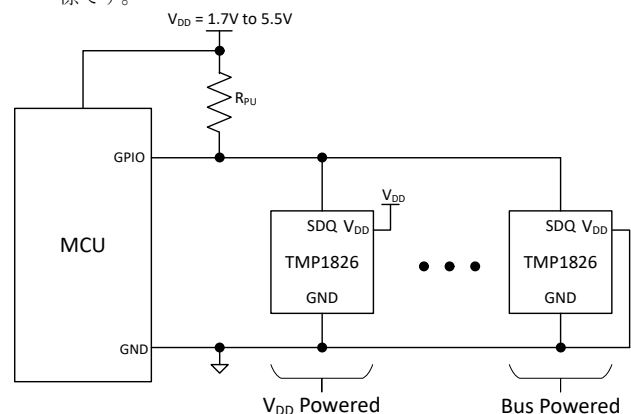
概略回路図
