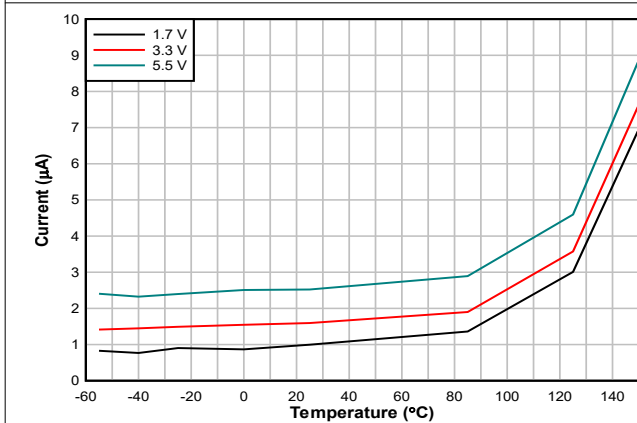
図 7-9. 温度変換電流と温度との関係
