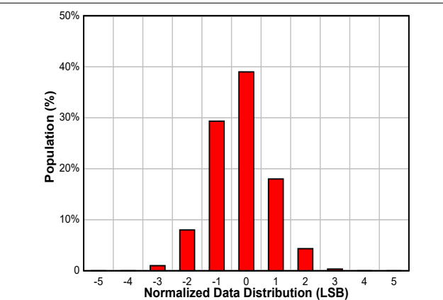
図 7-12. 変換時間 5.5ms、平均化オンでのデータの分散 (16 ビット・フォーマット)
