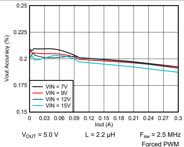
图 9-7. Output Voltage vs Output Current
