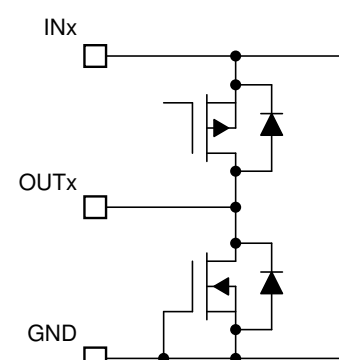
7-11. OUTx Pins
