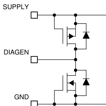
7-9. DIAGEN Pin
