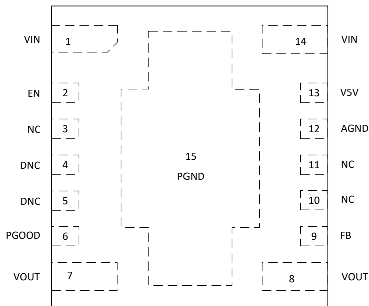
図 5-1. RDA Package 15-Pin QFN Top View
