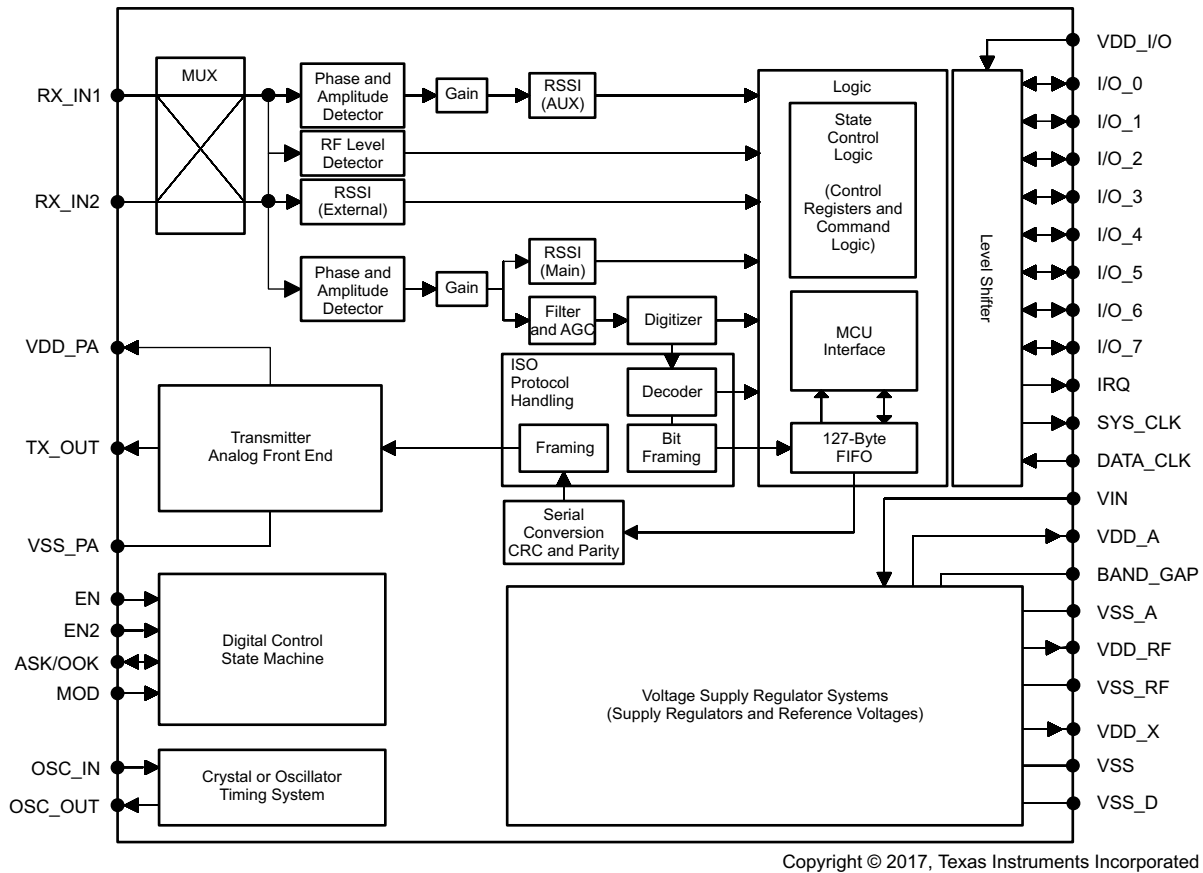
図 1-1. ブロック図
