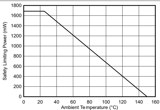
図 6-3. VDE に従って制限された電力の温度ディレーティング曲線、DWK パッケージ
