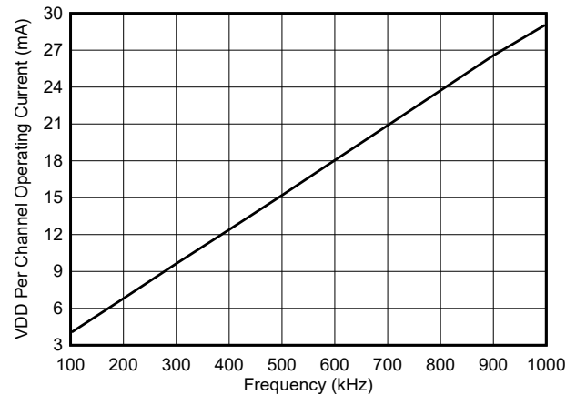
図 6-9. チャネルあたりの動作電流 ( I_{VDDA/B} ) と周波数との関係、 1.8\text{nF} 負荷
