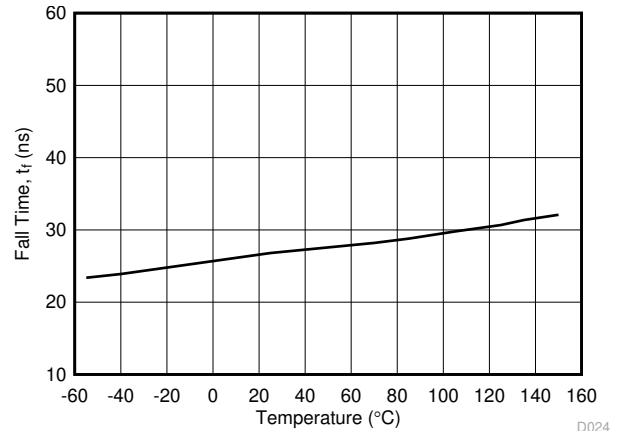
图 6-17. t_f Fall Time vs Temperature
