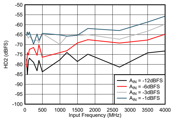
図 5-18. HD2 vs Input Frequency
