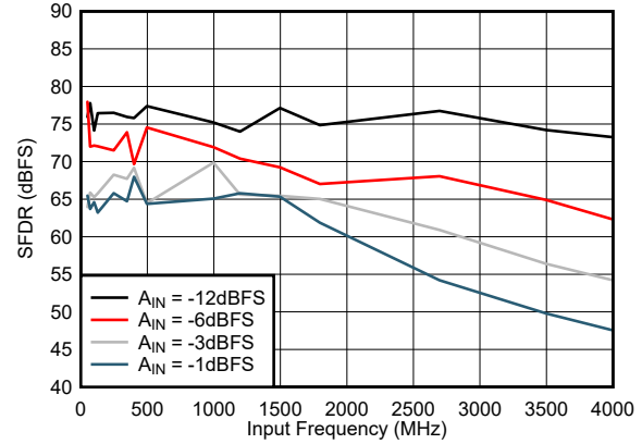
図 5-14. SFDR vs Input Frequency
