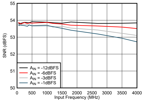
図 5-15. SNR vs Input Frequency
