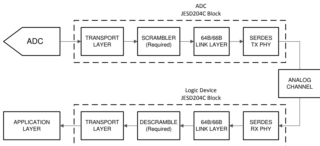
図 6-8. Simplified 64B/66B Encoded JESD204C Interface Diagram
