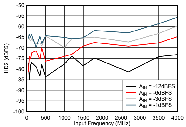
図 5-18. HD2 vs Input Frequency
