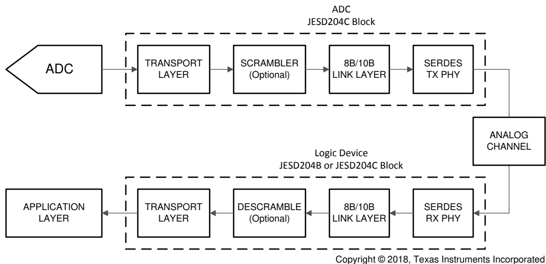
図 7-7. Simplified 8B/10B Encoded JESD204C Interface Diagram
