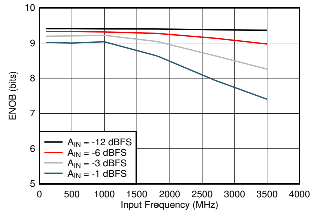
図 6-20. ENOB vs Input Frequency
