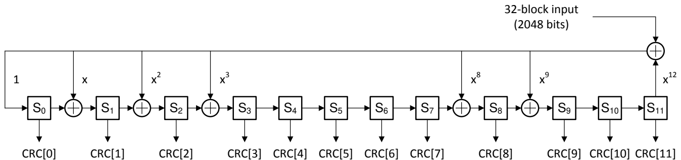
図 7-9. CRC-12 Parity Bit Generator
