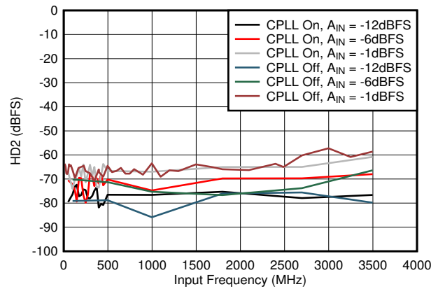
図 6-52. HD2 vs A_{IN} and C-PLL
