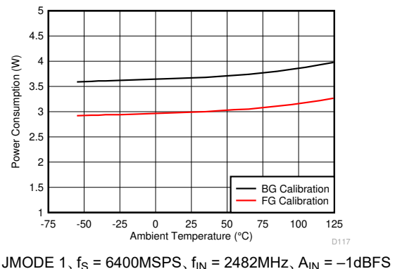
図 5-67. 消費電力と温度との関係
