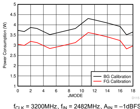
図 5-66. 消費電力と JMODE との関係
