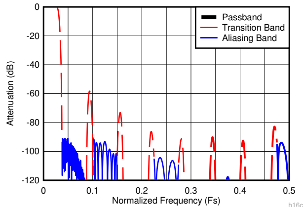
図 6-17. 16 倍デシメーション時の複合応答
