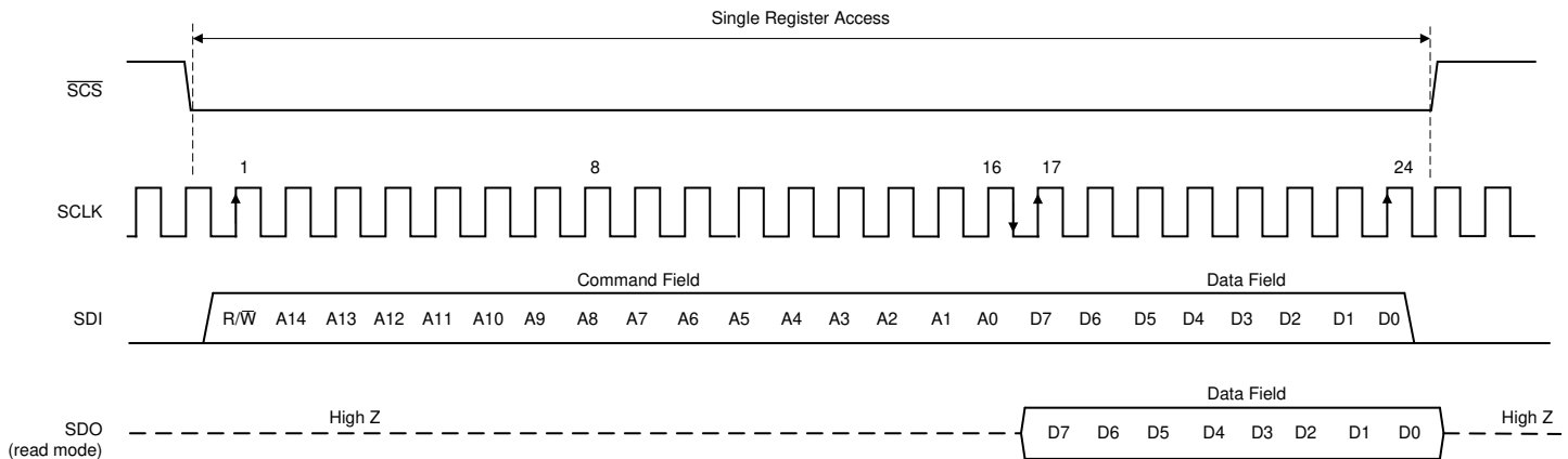
図 6-24. シリアル インターフェイス プロトコル : 単一読み取り / 書き込み
