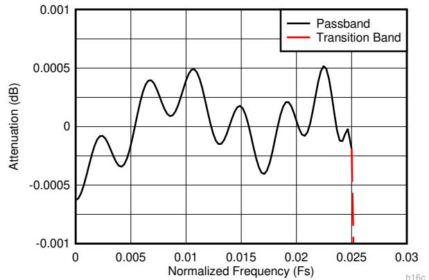
図 6-18. 16 倍デシメーション時の複合拡大パスバンド応答
