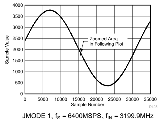
図 5-69. バックグラウンド キャリブレーション コアの遷移 (AC 信号)
