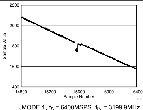
図 5-70. バックグラウンド キャリブレーション コアの遷移 (AC 信号の拡大)
