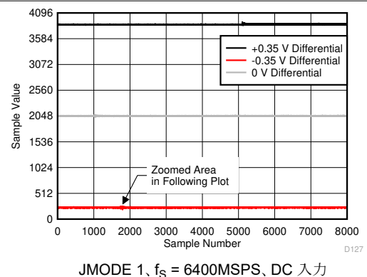
図 5-71. バックグラウンド キャリブレーション コアの遷移 (DC 信号)
