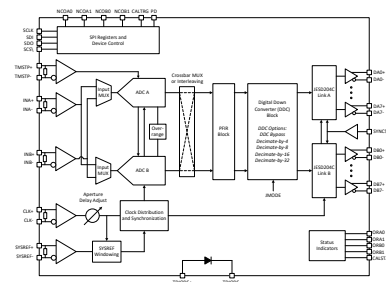
ADC12DJ4000RF ブロック図
