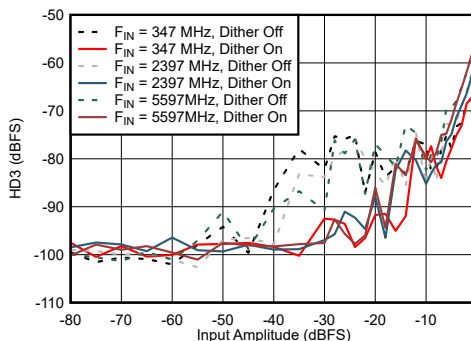
图 6-62. DES Mode: HD3 vs Input Amplitude and Dither
