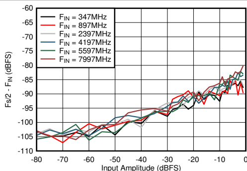
図 5-81. デュアル チャンネル モード : F_{\text{s}}/2 - F_{\text{IN}} と入力振幅および周波数との関係
