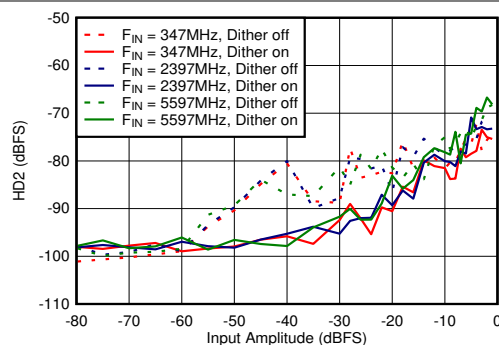
図 5-78. デュアル チャンネル モード : HD2 と入力振幅およびディザとの関係
