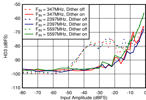
図 5-80. デュアル チャンネル モード : HD3 と入力振幅およびディザとの関係
