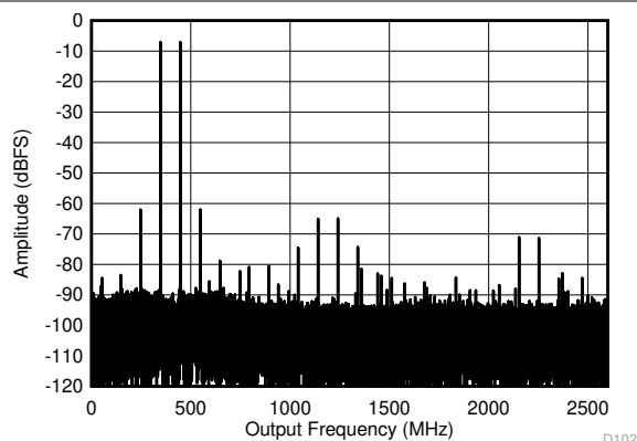
図 5-27. デュアルチャネルモード：5597MHz での 2 トーン FFT
