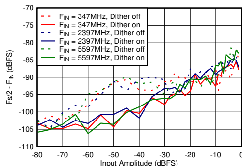
図 5-82. デュアル チャンネル モード : F_{\text{s}}/2 - F_{\text{IN}} と入力振幅およびディザとの関係
