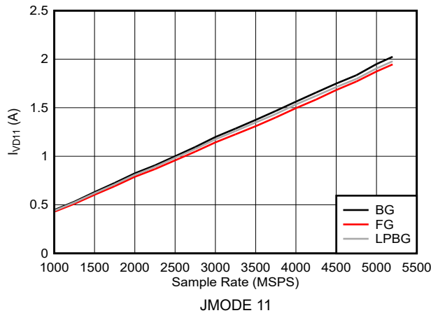
図 6-151. デュアルチャネルモード: I_{VD11} とサンプルレートとの関係 (ADC12DJ5210RF)
