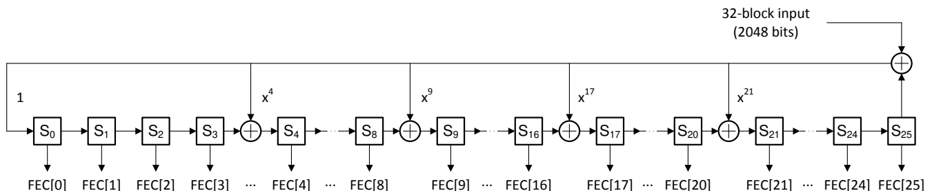
図 7-22. FEC パリティビットジェネレータ
