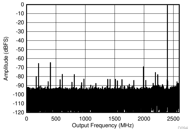
図 6-19. デュアル チャネル モード : 2397MHz でのシングル トーン FFT
