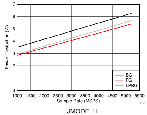
図 6-160. デュアルチャネル モード：消費電力とサンプル レートとの関係
