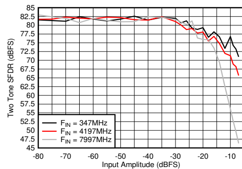
図 6-108. デュアルチャネルモード：2 トーン SFDR と入力振幅との関係
