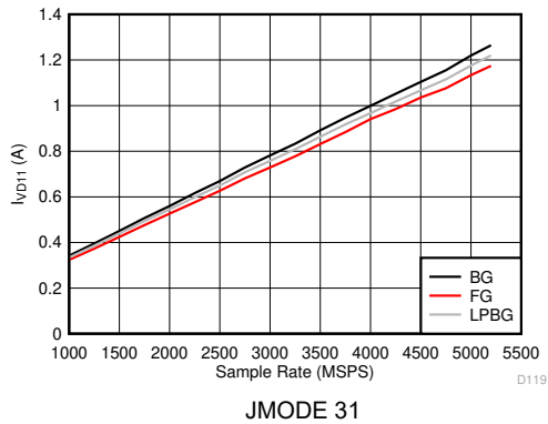
図 6-153. デュアルチャネルモード: I_{VD11} とサンプルレートとの関係 (ADC12DJ5200RF)
