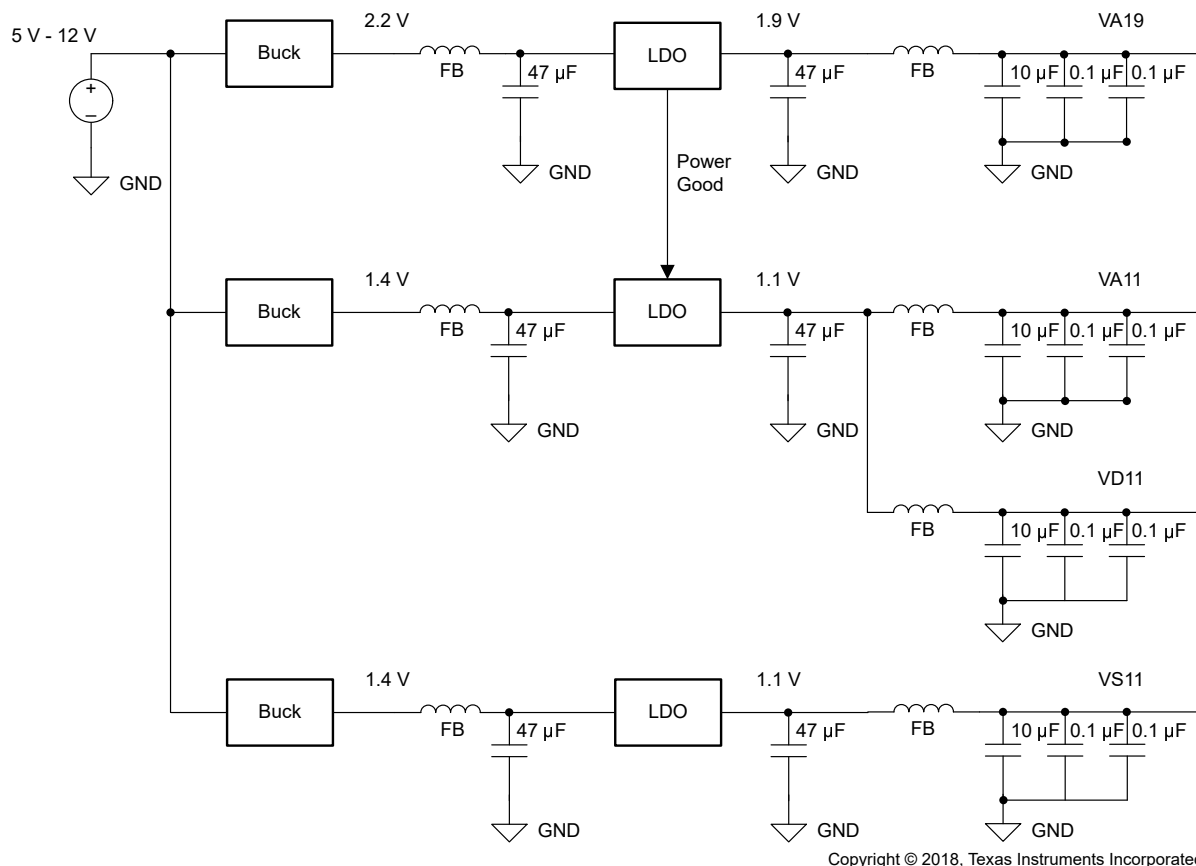
図 8-15. LDO リニア レギュレータのアプローチ例 (ADC12DJ5210RF)
