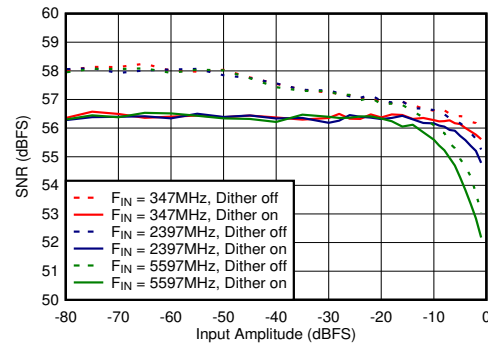
図 6-72. デュアル チャネル モード : SNR と入力振幅およびディザとの関係
