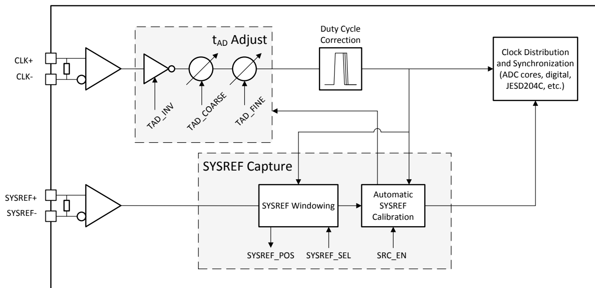
図 7-2. クロッキング サブシステム
