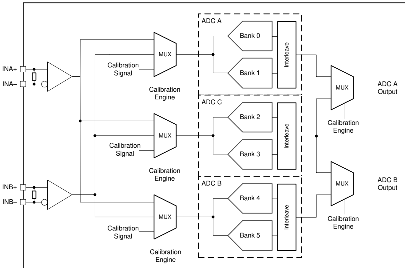
図 7-26. ADC12DJ52x0RF キャリブレーション システム ブロック図
