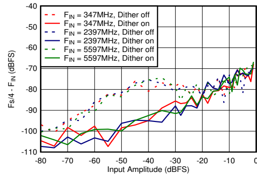
図 6-70. DES モード : F_s/4 - F_{\text{IN}} と入力振幅およびディザとの関係
