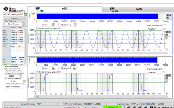
図 8-11. 5GSPS シングル チャネル オシロスコープにおける 200MHz、正弦波 (チャネル A) および 40MHz、方形波 (チャネル B) 時間ドメイン
