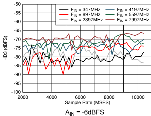
図 6-39. DES モード: HD3 とサンプル レートおよび入力周波数との関係
