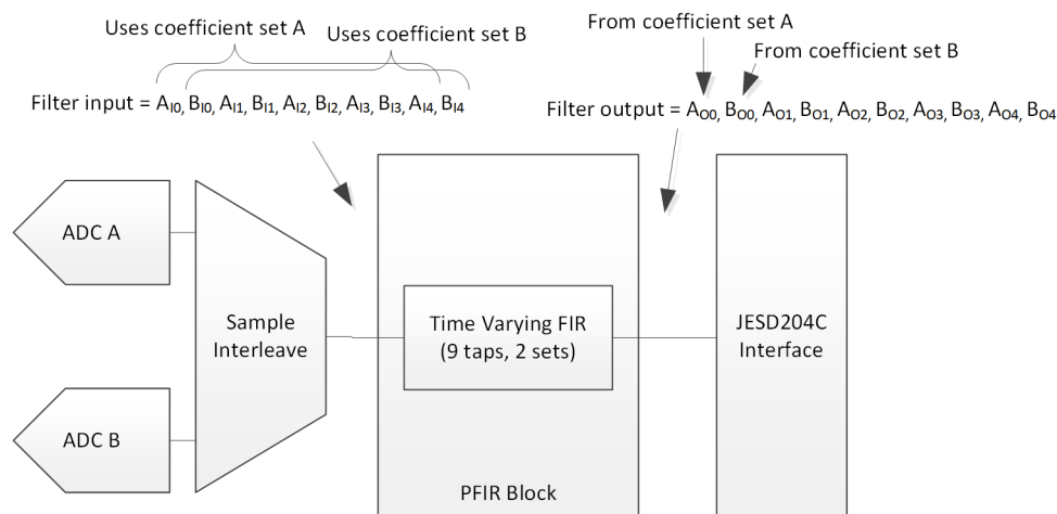
図 7-6. 時変フィルタ PFIR のブロック図
