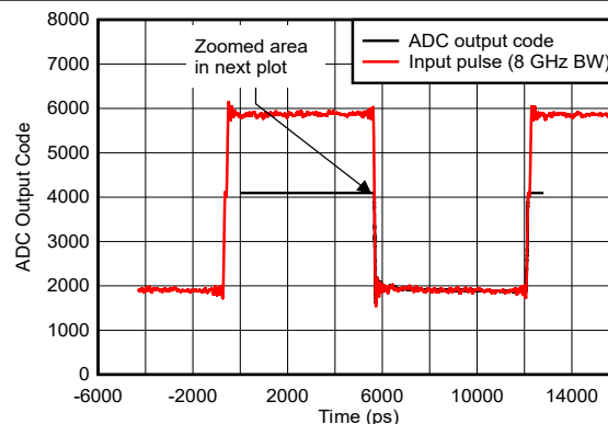
図 6-168. パルス オーバードライブ 回復
