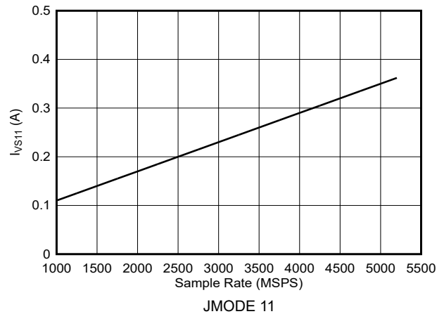
図 6-152. デュアルチャネルモード: I_{VS11} とサンプルレートとの関係 (ADC12DJ5210RF)
