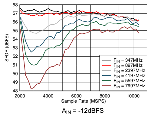
図 6-34. DES モード: SFDR とサンプル レートおよび入力周波数との関係
