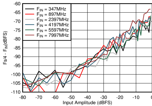
図 6-69. DES モード : F_s/4 - F_{\text{IN}} と入力振幅および周波数との関係
