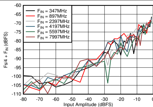
図 6-67. DES モード : F_s/4 + F_{\text{IN}} と入力振幅および周波数との関係
