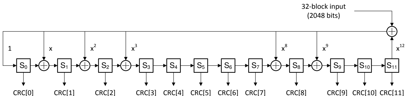
図 7-21. CRC-12 パリティビットジェネレータ
