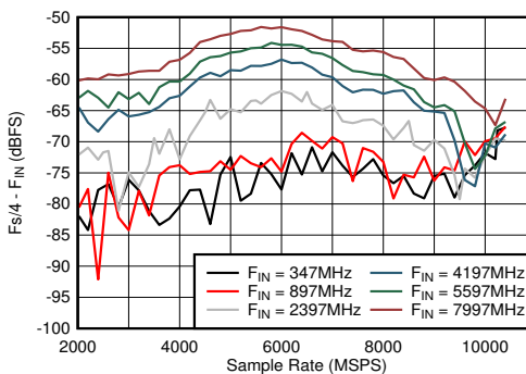
図 6-43. DES モード : F_s/4 - F_{IN} とサンプル レートおよび入力周波数との関係
