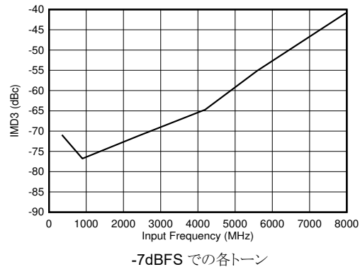
図 6-104. デュアルチャネルモード : IMD3 と入力周波数との関係
