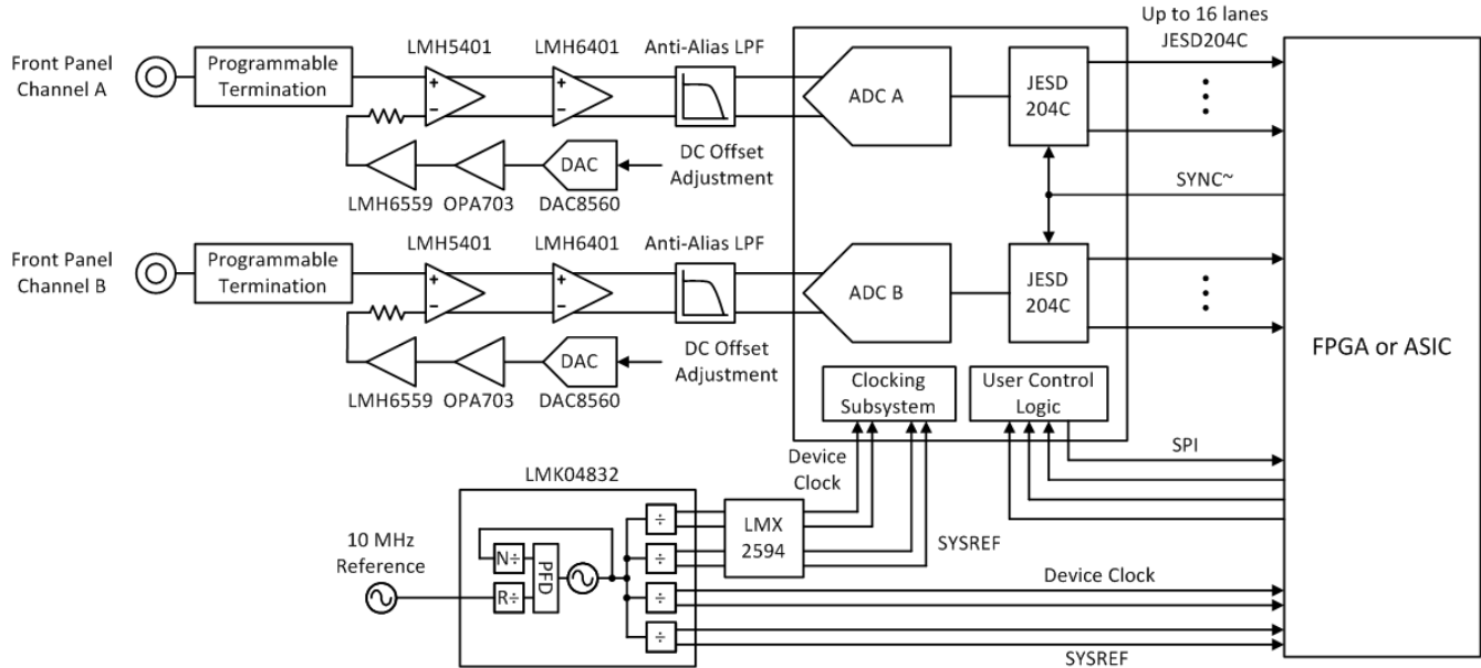
図 8-5. 再構成可能オシロスコープの標準構成
