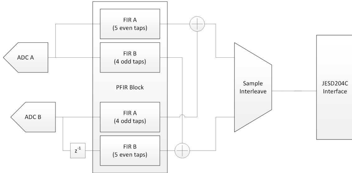
図 7-7. 代替 I/Q 補正タイプ フィルタのブロック図
