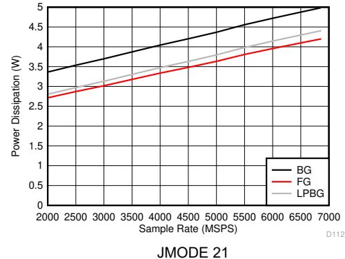
図 6-142. DES モード : 消費電力とサンプル レートとの関係
