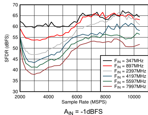
図 6-32. DES モード: SFDR とサンプル レートおよび入力周波数との関係
