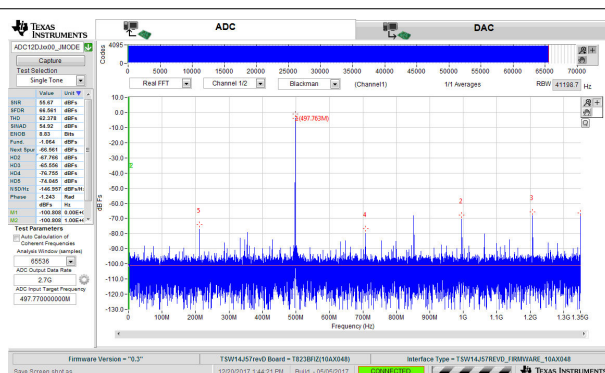
図 8-3. 497.77MHz 入力信号用 FFT、2.7GSPS、JMODE2
