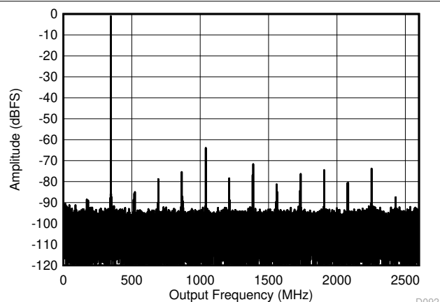
図 6-17. デュアルチャネル モード : 347MHz でのシングル トーン FFT
