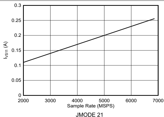
図 6-134. DES モード : I_{VS11} とサンプル レートとの関係 (ADC12DJ5210RF)
