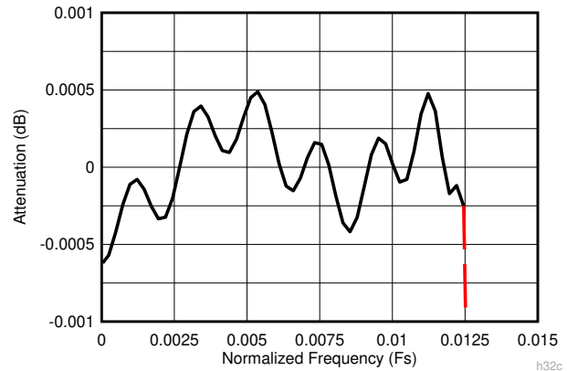
図 7-18. 32 倍デシメーション時の複合拡大パスバンド応答
