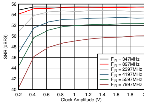
図 6-81. DES モード : SNR とクロック振幅との関係
