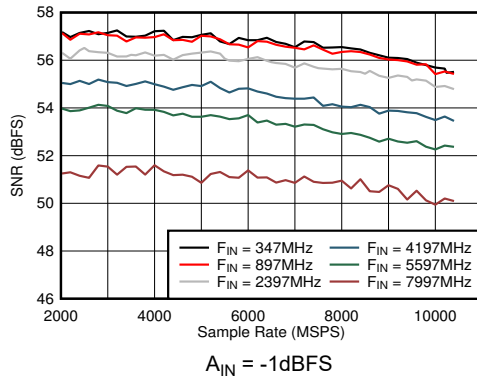
図 6-29. DES モード:SNR とサンプル レートおよび入力周波数との関係
