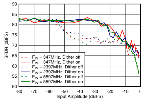
図 6-74. デュアル チャネル モード : SFDR と入力振幅およびディザとの関係
