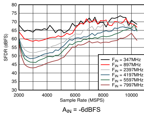
図 6-33. DES モード: SFDR とサンプル レートおよび入力周波数との関係
