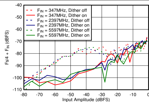
図 6-68. DES モード : F_s/4 + F_{\text{IN}} と入力振幅およびディザとの関係
