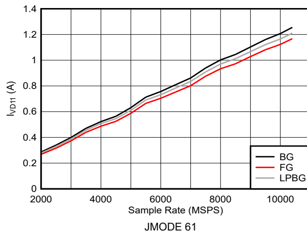
図 6-139. DES モード : I_{VD11} とサンプル レートとの関係 (ADC12DJ5210RF)
