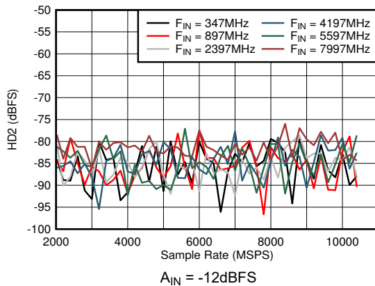
図 6-37. DES モード: HD2 とサンプル レートおよび入力周波数との関係
