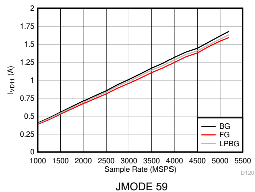
図 6-156. デュアルチャネルモード: I_{VD11} とサンプルレートとの関係 (ADC12DJ5200RF)
