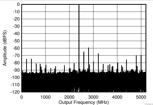
図 6-7. DES モード : 2397MHz でのシングル トーン FFT
