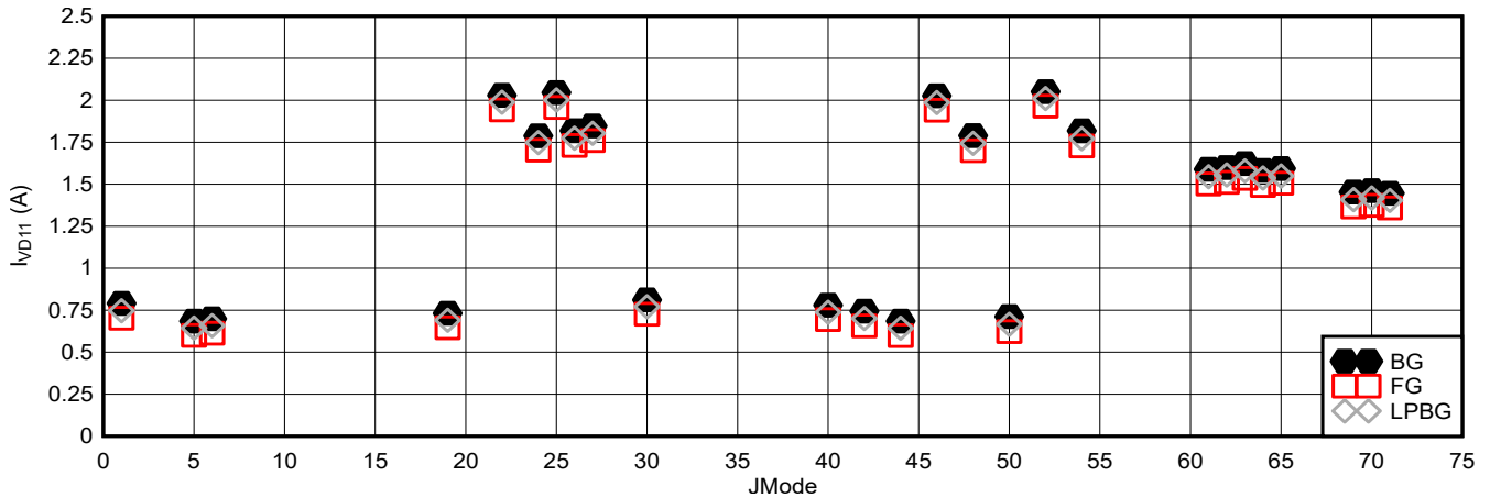
図 6-111. DES モード : I_{VD11} と JMODE (10.4GSPS) との関係 (ADC12DJ5200RF)
