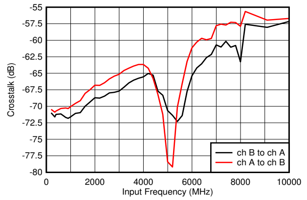
図 6-2. クロストークと入力周波数との関係
