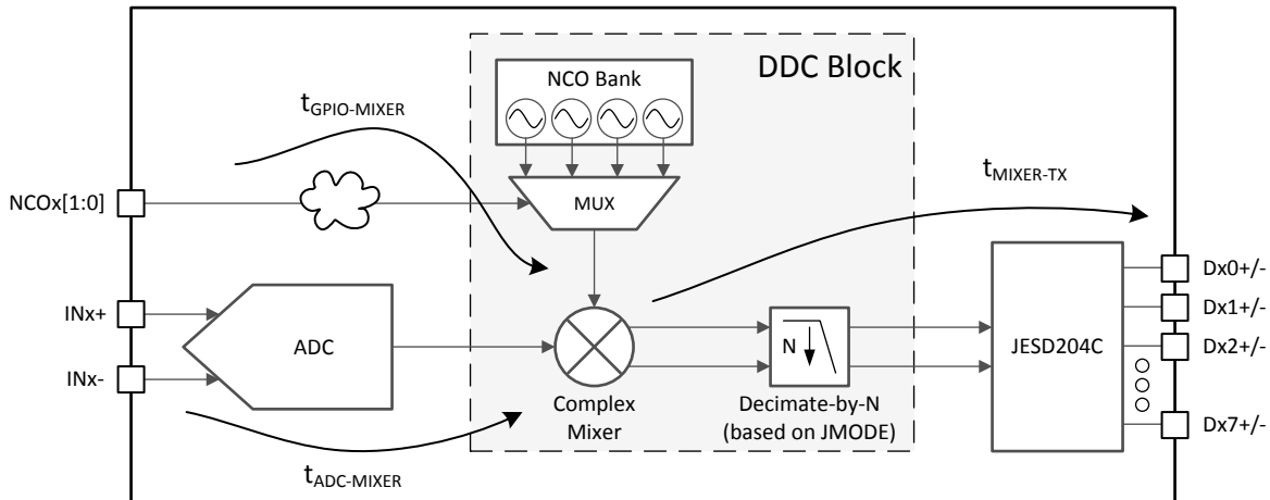
図 7-10. NCO 高速周波数ホッピングのレイテンシ図
