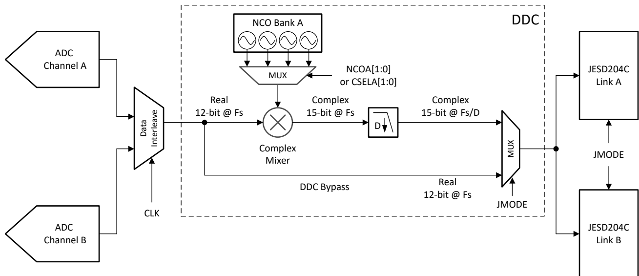
図 7-9. シングルチャネルモードでのデジタルダウンコンバージョンブロック
