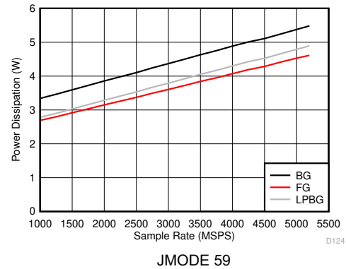
図 6-162. デュアルチャネル モード：消費電力とサンプル レートとの関係
