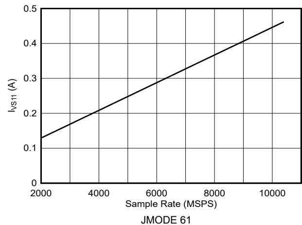
図 6-140. DES モード : I_{VS11} とサンプル レートとの関係 (ADC12DJ5210RF)
