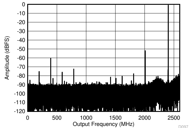
図 6-22. デュアル チャネル モード : 7997MHz でのシングル トーン FFT
