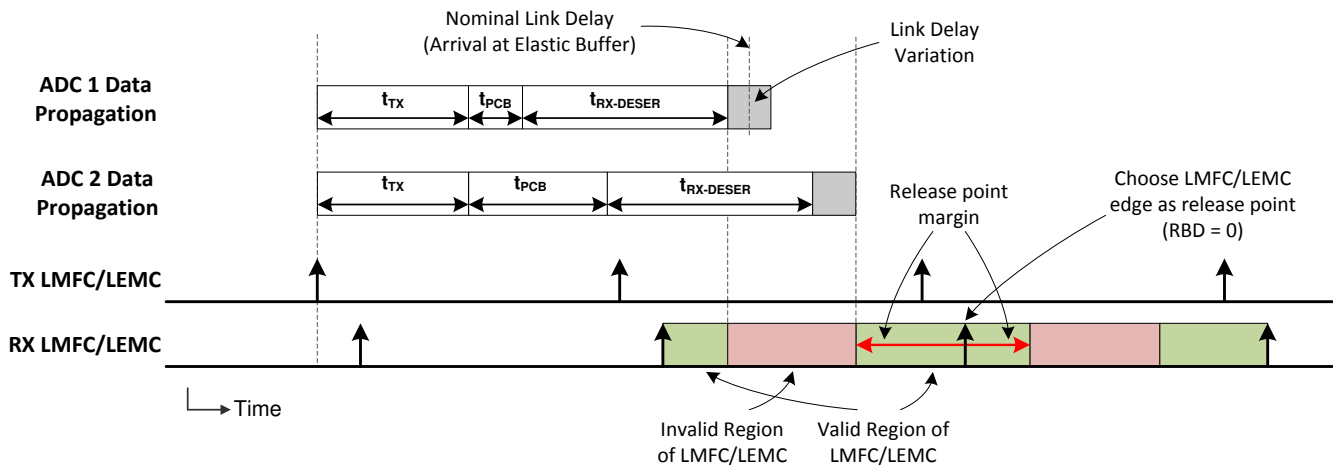
図 7-23. 弾性バッファリリースポイント選択のための LMFC/LEMC 有効領域定義
