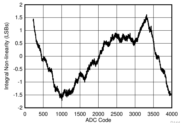
図 6-4. INL と ADC コードとの関係
