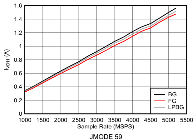
図 6-157. デュアルチャネルモード: I_{VD11} とサンプルレートとの関係 (ADC12DJ5210RF)
