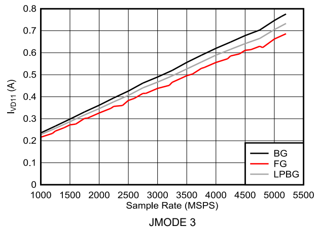
図 6-148. デュアル チャネル モード: I_{VD11} とサンプル レートとの関係 (ADC12DJ5210RF)
