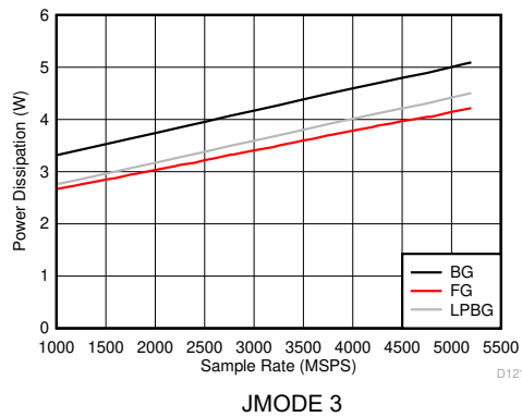
図 6-159. デュアルチャネル モード：消費電力とサンプル レートとの関係
