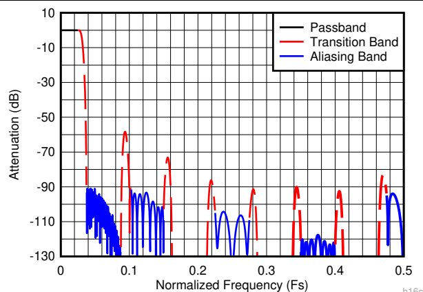
図 7-15. 16 倍デシメーション時の複合応答
