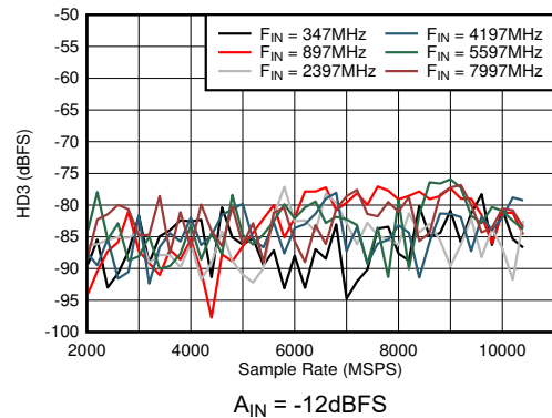
図 6-40. DES モード: HD3 とサンプル レートおよび入力周波数との関係
