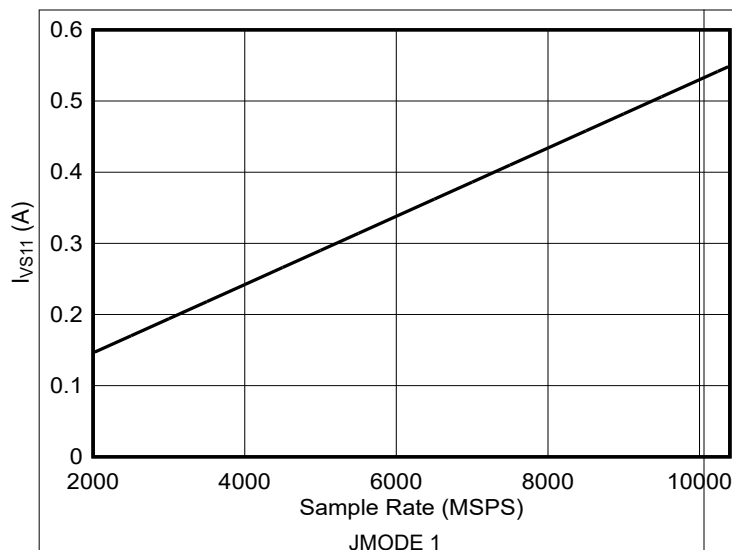
図 6-131. DES モード : I_{VS11} とサンプル レートとの関係 (ADC12DJ5210RF)
