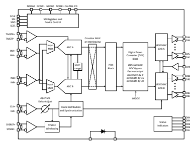
ADC12DJ52x0RF ブロック図
