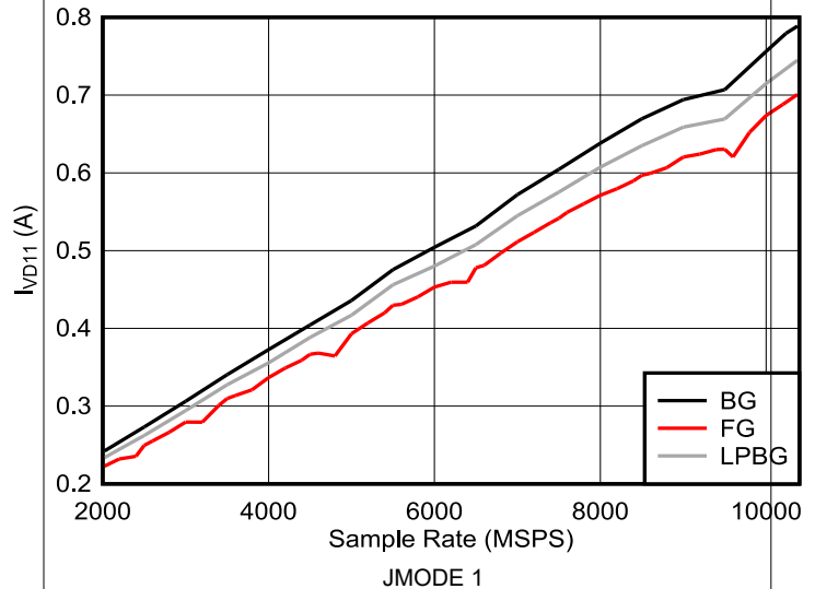
図 6-130. DES モード : I_{VD11} とサンプル レートとの関係 (ADC12DJ5210RF)
