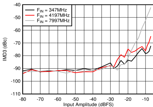
図 6-105. デュアルチャネルモード : IMD3 と入力振幅との関係
