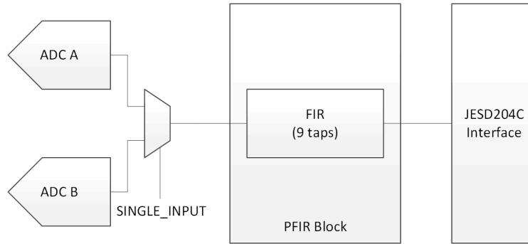
図 7-5. シングル チャネル イコライゼーション PFIR のブロック図
