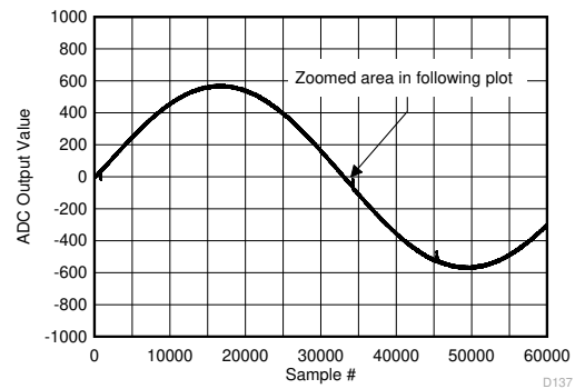
図 6-164. バックグラウンドキャリブレーションコア遷移 (AC 信号)
