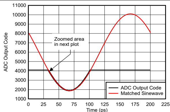
図 6-170. 正弦波オーバードライブ回復
