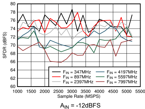
図 6-49. デュアル チャネル モード: SFDR とサンプル レートおよび入力周波数との関係
