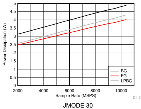
図 6-143. DES モード : 消費電力とサンプル レートとの関係
