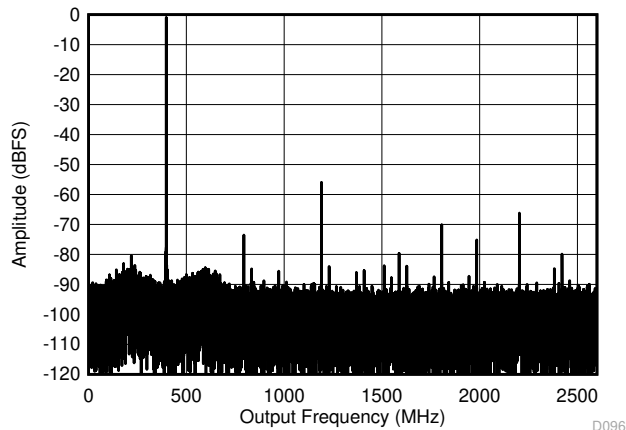
図 6-21. デュアル チャネル モード : 5597MHz でのシングル トーン FFT
