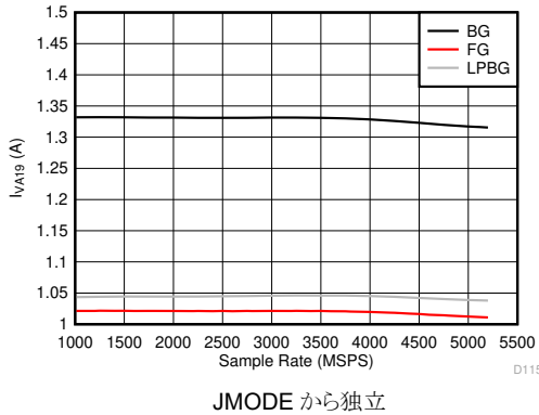
図 6-145. デュアル チャネル モード : I_{VA19} とサンプル レートとの関係
