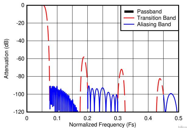
図 7-13. 8 倍デシメーション時の複合応答
