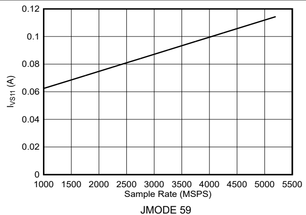
図 6-158. デュアルチャネルモード: I_{VS11} とサンプルレートとの関係 (ADC12DJ5210RF)
