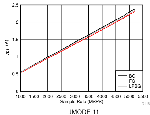
図 6-150. デュアル チャネル モード: I_{VD11} とサンプル レートとの関係 (ADC12DJ5200RF)
