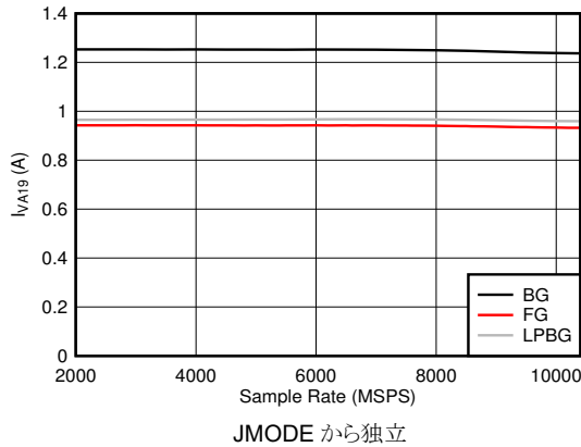
図 6-127. DES モード : I_{VA19} とサンプル レートとの関係
