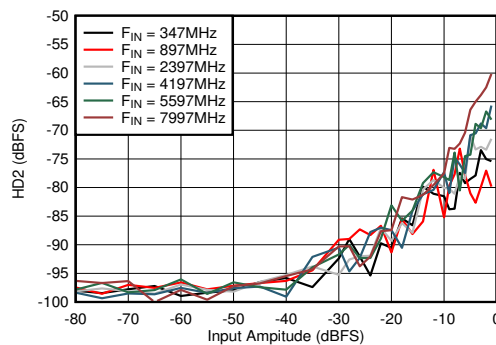
図 6-75. デュアル チャネル モード : HD2 と入力振幅および周波数との関係
