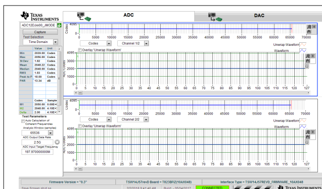
図 8-10. 2.5GSPS デュアル チャネル オシロスコープにおけるアイドルチャネル ノイズ (入力なし)
