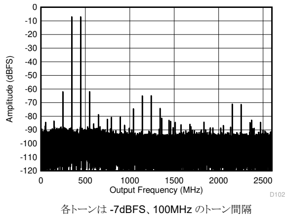
図 6-27. デュアルチャネルモード：2 トーン FFT (5597MHz で)
