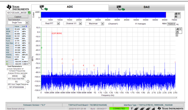
図 8-9. 5GSPS シングル チャネル オシロスコープにおける 200MHz、正弦波周波数ドメイン (FFT)
