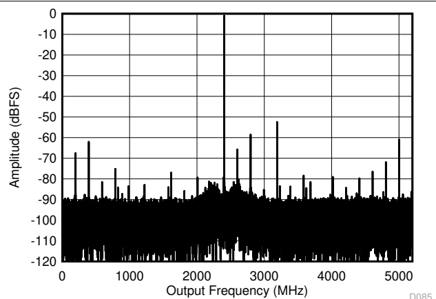
図 6-10. DES モード : 7997MHz でのシングル トーン FFT
