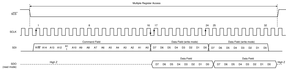
図 7-28. シリアル インターフェイス プロトコル : ストリーミング読み取り/書き込み
