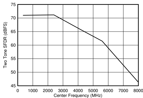
図 6-107. デュアルチャネルモード：2 トーン SFDR と入力周波数との関係
