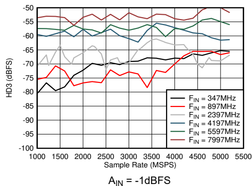
図 6-53. デュアル チャネル モード : HD3 とサンプル レートおよび入力周波数との関係
