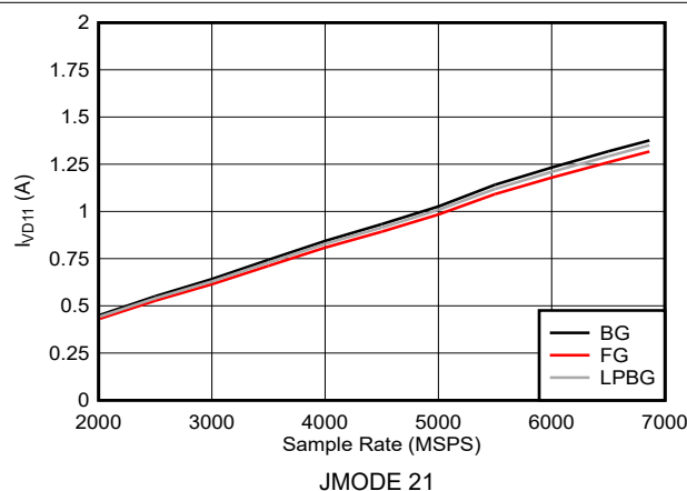
図 6-133. DES モード : I_{VD11} とサンプル レートとの関係 (ADC12DJ5210RF)
