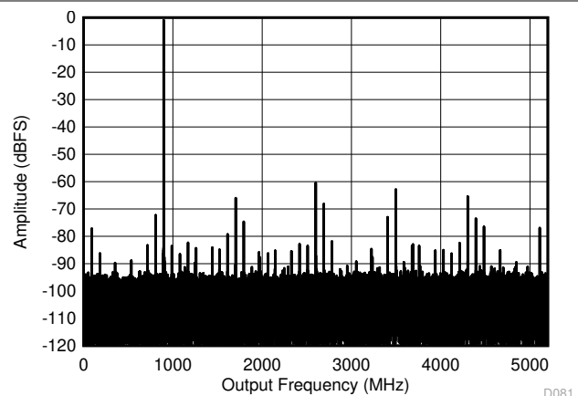
図 6-6. DES モード : 897MHz でのシングル トーン FFT
