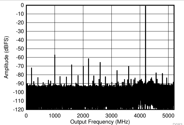
図 6-8. DES モード : 4197MHz でのシングル トーン FFT
