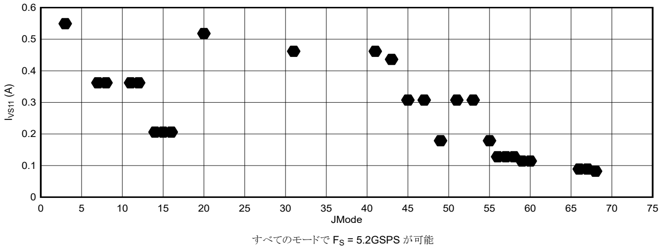
図 6-119. デュアル チャネル モード : I_{VS11} と JMODE (5.2GSPS) との関係 (ADC12DJ5210RF)
