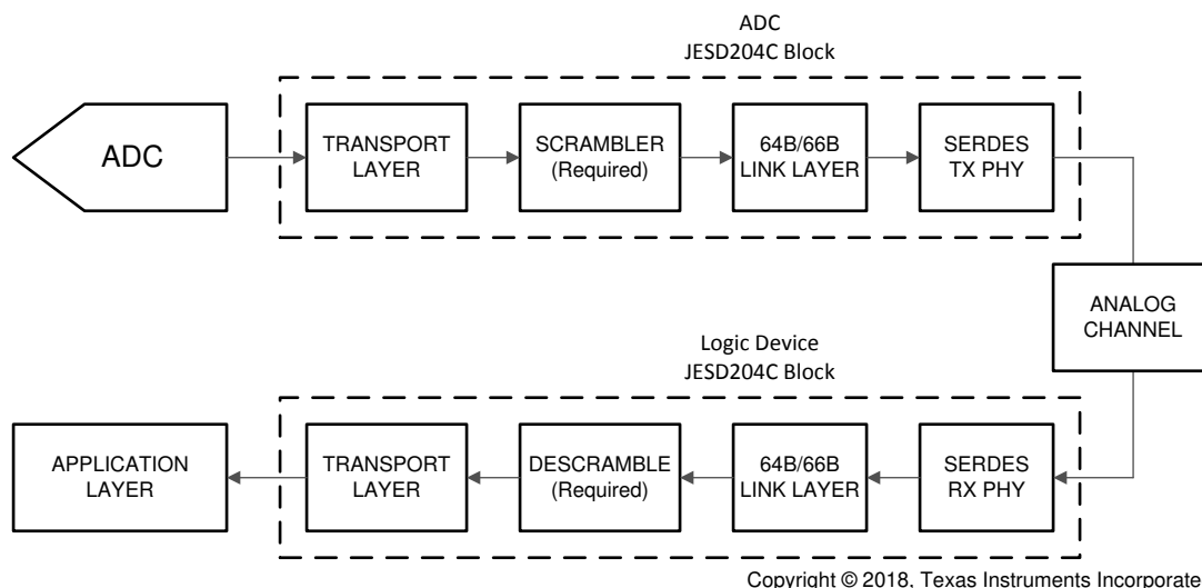
図 7-20. 64B/66B エンコードされた JESD204C インターフェイスのダイアグラム
