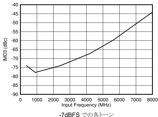
図 6-99. DES モード : IMD3 と入力周波数との関係
