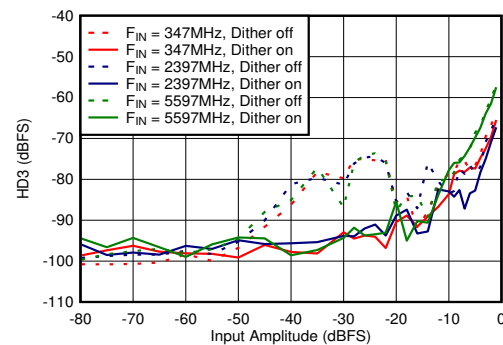
図 6-64. DES モード : HD3 と入力振幅およびディザとの関係
