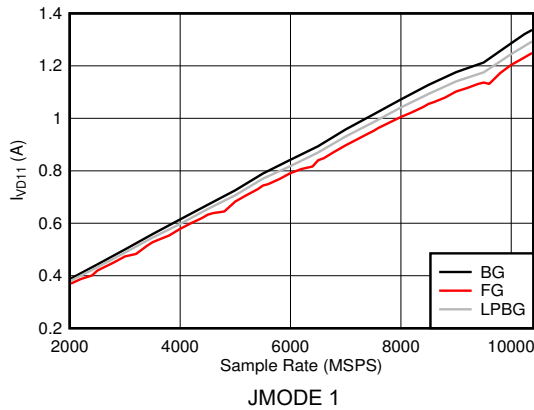
図 6-129. DES モード : I_{VD11} とサンプル レートとの関係 (ADC12DJ5200RF)
