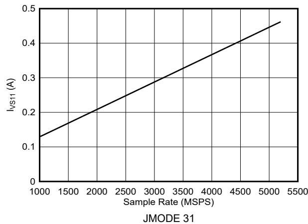
図 6-155. デュアルチャネルモード: I_{VS11} とサンプルレートとの関係 (ADC12DJ5210RF)
