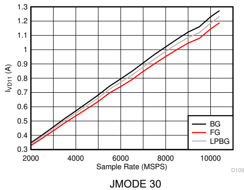
図 6-135. DES モード : I_{VD11} とサンプル レートとの関係 (ADC12DJ5200RF)
