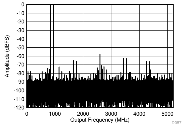
図 6-12. DES モード : 2 トーン FFT (897MHz で)
