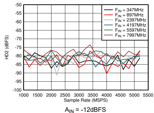
図 6-52. デュアル チャネル モード : HD2 とサンプル レートおよび入力周波数との関係
