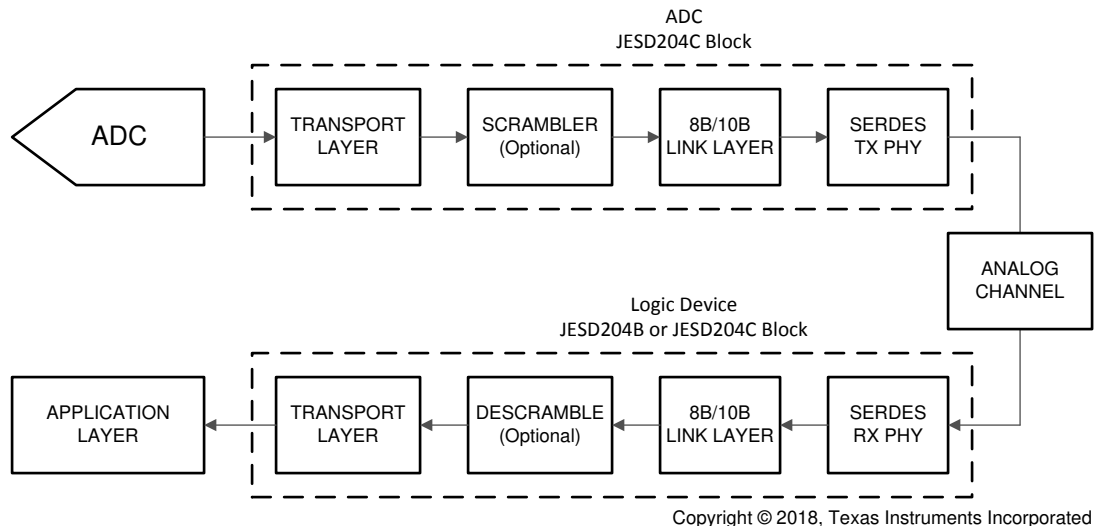
図 7-19. 8B/10B エンコードされた JESD204C インターフェイスのダイアグラム
