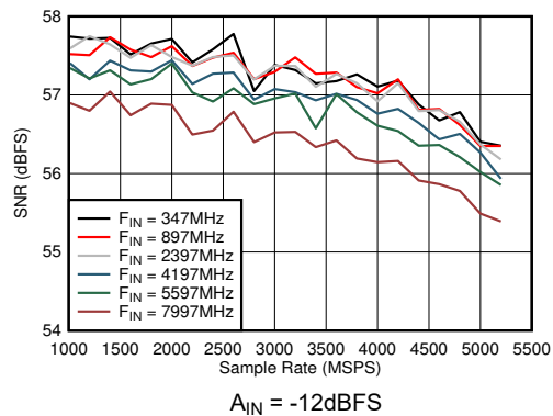
図 6-46. デュアル チャネル モード : SNR とサンプル レートおよび入力周波数との関係
