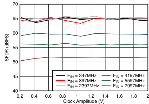
図 6-84. デュアル チャネル モード : SFDR とクロック振幅との関係
