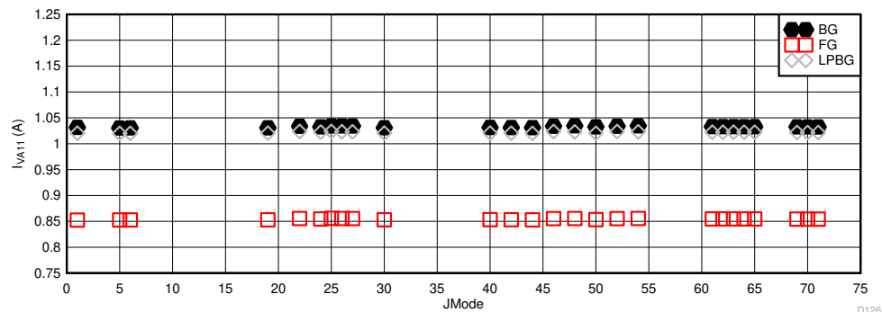
図 6-109. DES モード： I_{VA19} と JMODE (10.4GSPS) との関係
