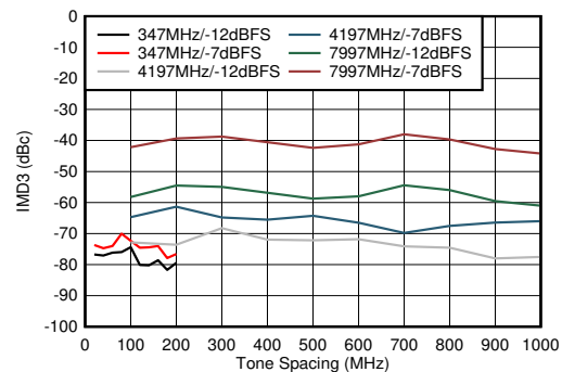
図 6-106. デュアルチャネルモード : IMD3 とトーン間隔との関係
