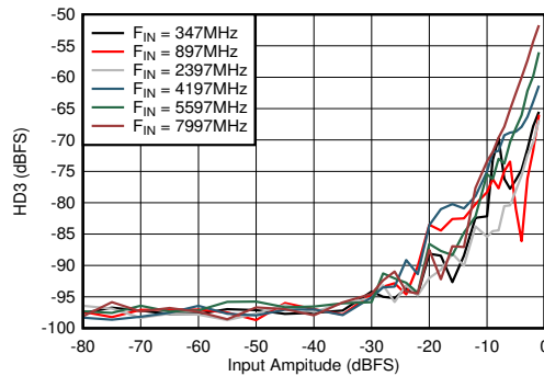
図 6-77. デュアル チャネル モード : HD3 と入力振幅および周波数との関係
