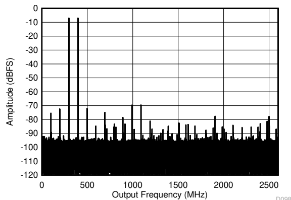
図 6-23. デュアルチャネルモード：2 トーン FFT (347MHz で)
