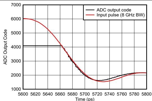
図 6-169. パルスオーバードライブ回復の拡大図
