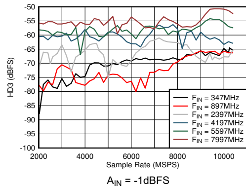
図 6-38. DES モード: HD3 とサンプル レートおよび入力周波数との関係
