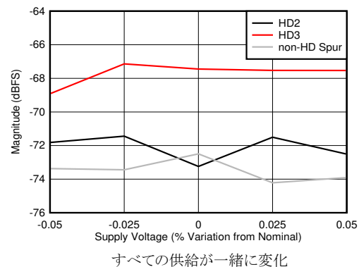
図 6-96. デュアル チャネル モード : HD2、HD3、およびワーストケースの非 HD スプリアスと電源電圧との関係
