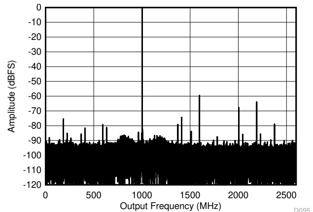
図 6-20. デュアル チャネル モード : 4197MHz でのシングル トーン FFT
