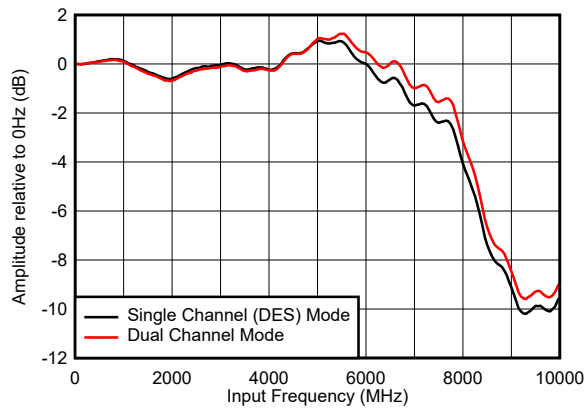
図 6-1. 入力振幅と入力周波数との関係
