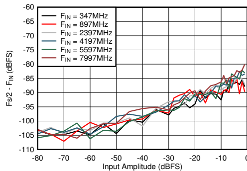
図 6-79. デュアル チャネル モード : F_{\text{s}}/2 - F_{\text{IN}} と入力振幅および周波数との関係
