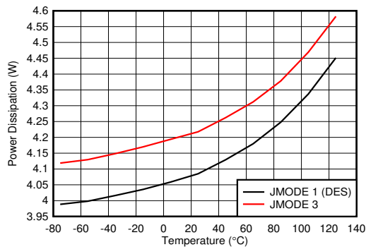
図 6-163. 消費電力と温度との関係
