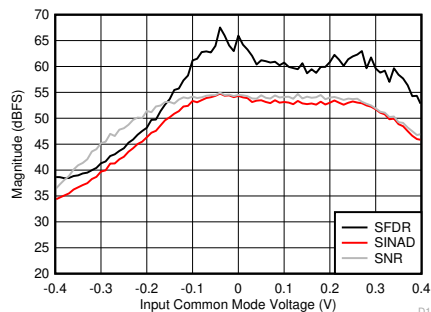
図 6-97. SNR、SFDR、SINAD と入力同相電圧との関係
