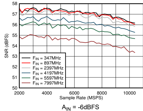
図 6-30. DES モード:SNR とサンプル レートおよび入力周波数との関係
