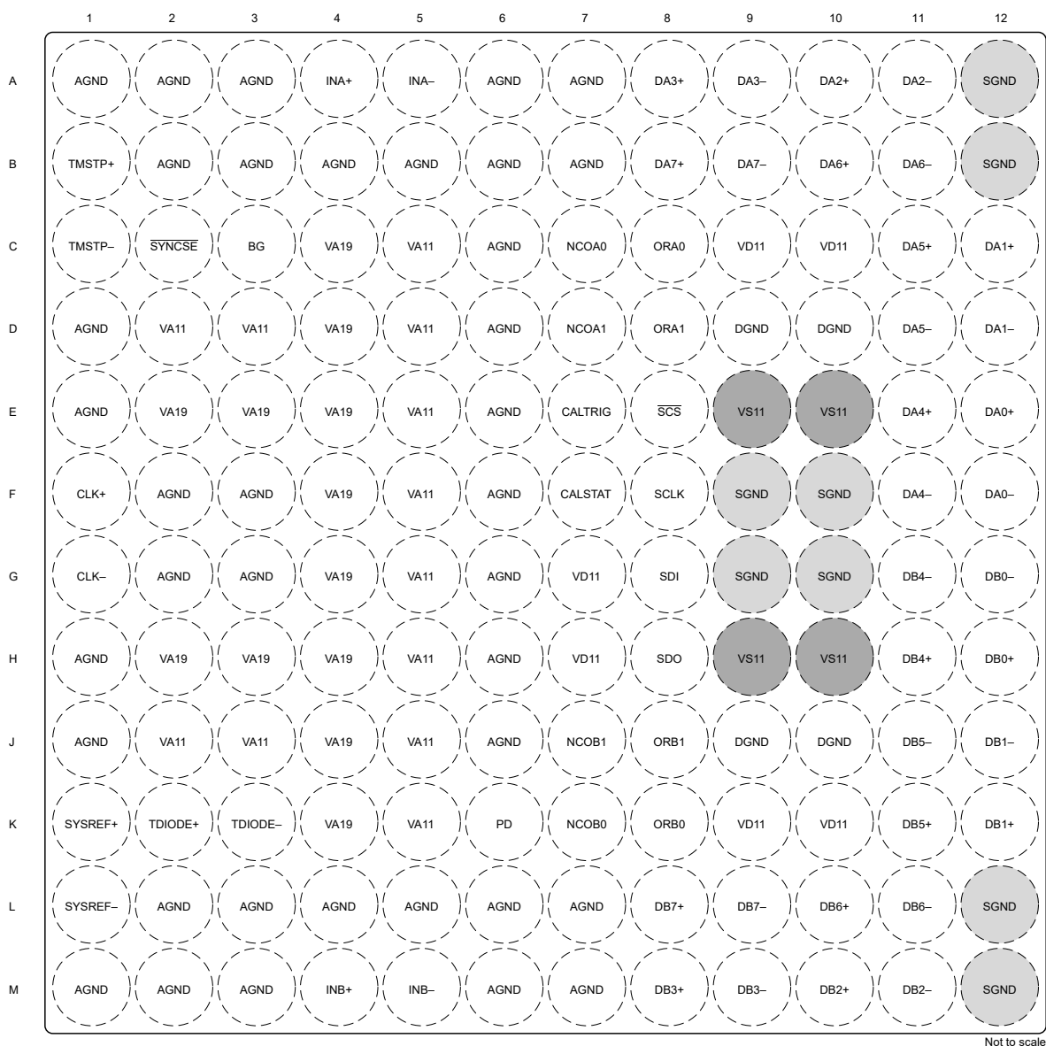
図 5-2. ADC12DJ5210RF AAV パッケージ、144 ボール フリップ チップ BGA (上面図)
