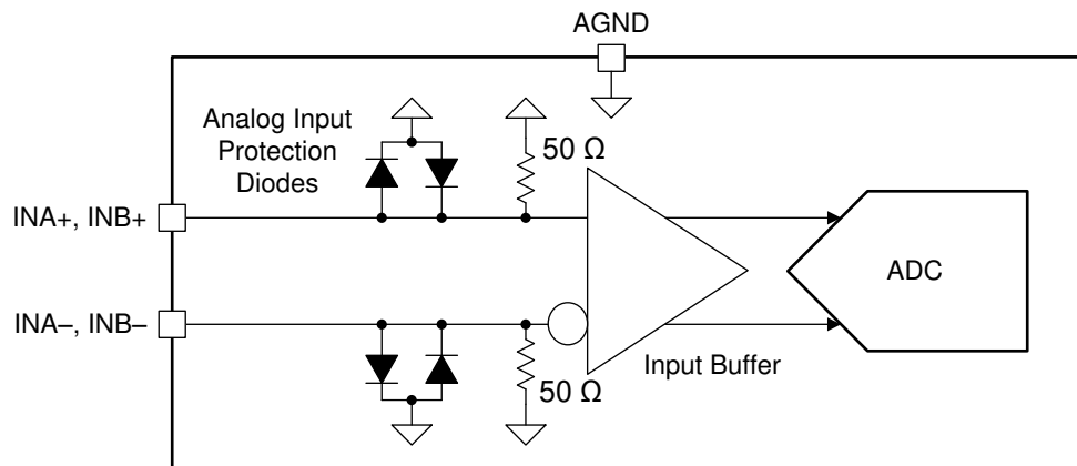
図 7-1. ADC12DJ52x0RF アナログ入力内部終端および保護図
