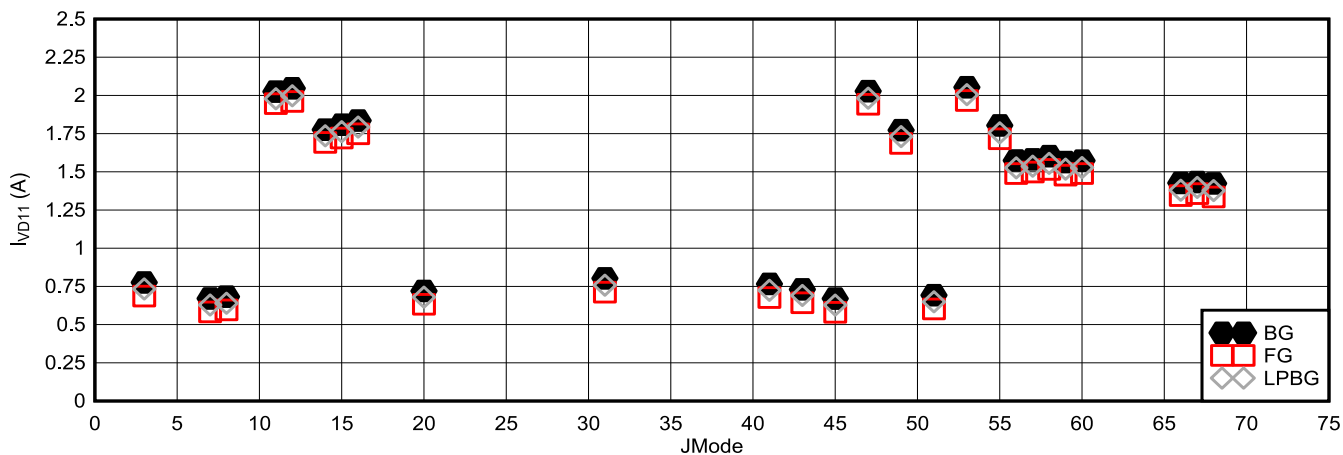
図 6-117. デュアル チャネル モード : I_{VD11} と JMODE (5.2GSPS) との関係 (ADC12DJ5200RF)
