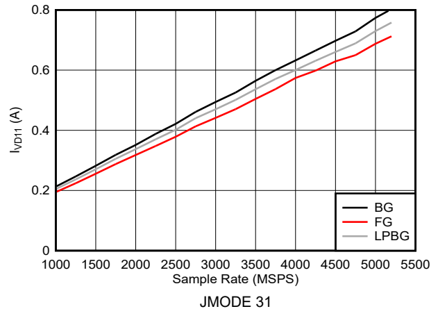
図 6-154. デュアルチャネルモード: I_{VD11} とサンプルレートとの関係 (ADC12DJ5210RF)
