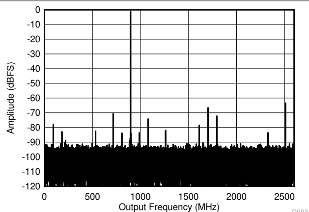
図 6-18. デュアルチャネル モード : 897MHz でのシングル トーン FFT
