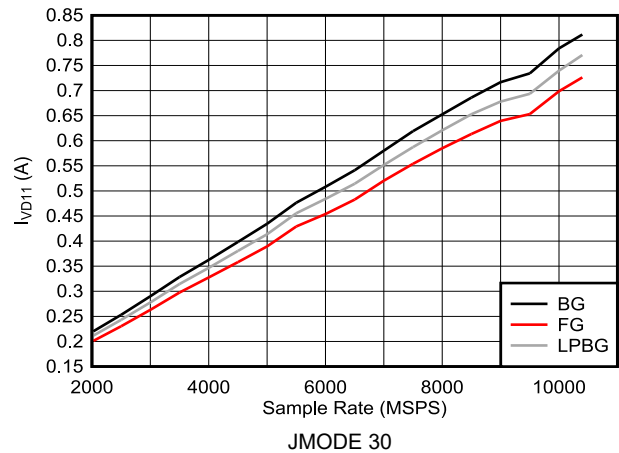
図 6-136. DES モード : I_{VD11} とサンプル レートとの関係 (ADC12DJ5210RF)
