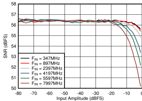
図 6-71. デュアル チャネル モード : SNR と入力振幅および周波数との関係
