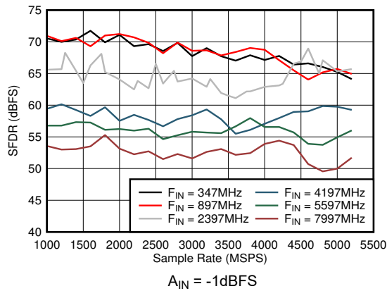
図 6-47. デュアル チャネル モード: SFDR とサンプル レートおよび入力周波数との関係
