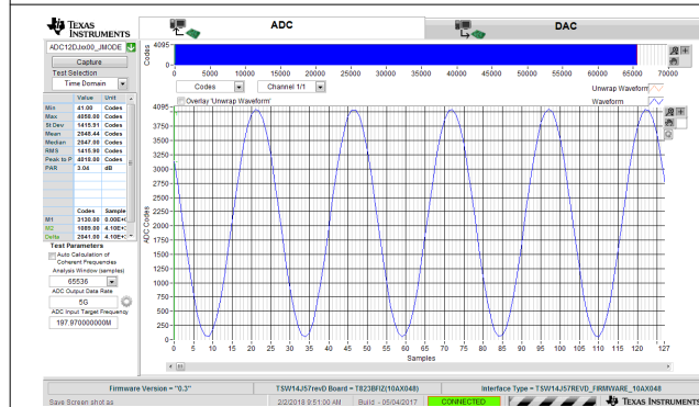
図 8-8. 5GSPS シングル チャネル オシロスコープにおける 200MHz、正弦波時間ドメイン
