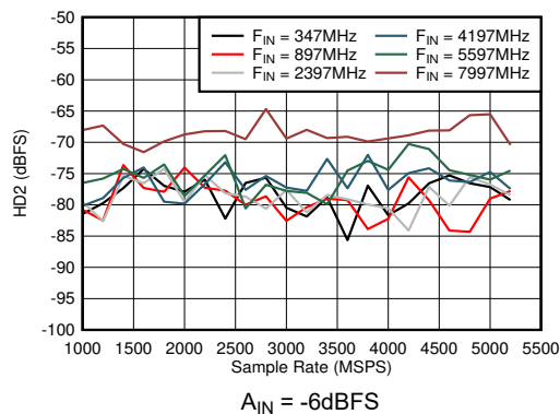
図 6-51. デュアル チャネル モード : HD2 とサンプル レートおよび入力周波数との関係
