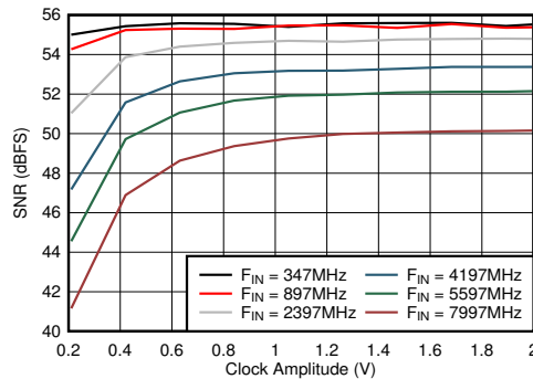
図 6-83. デュアル チャネル モード : SNR とクロック振幅との関係
