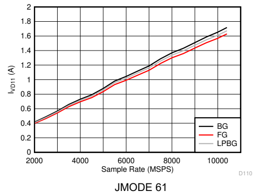
図 6-138. DES モード : I_{VD11} とサンプル レートとの関係 (ADC12DJ5200RF)
