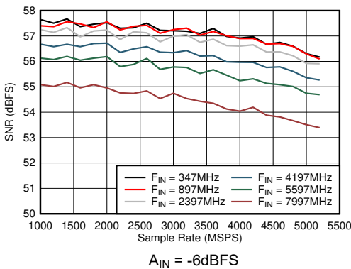
図 6-45. デュアル チャネル モード : SNR とサンプル レートおよび入力周波数との関係
