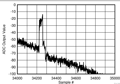
図 6-165. バックグラウンド キャリブレーション コアの遷移 (AC 信号 - 拡大)
