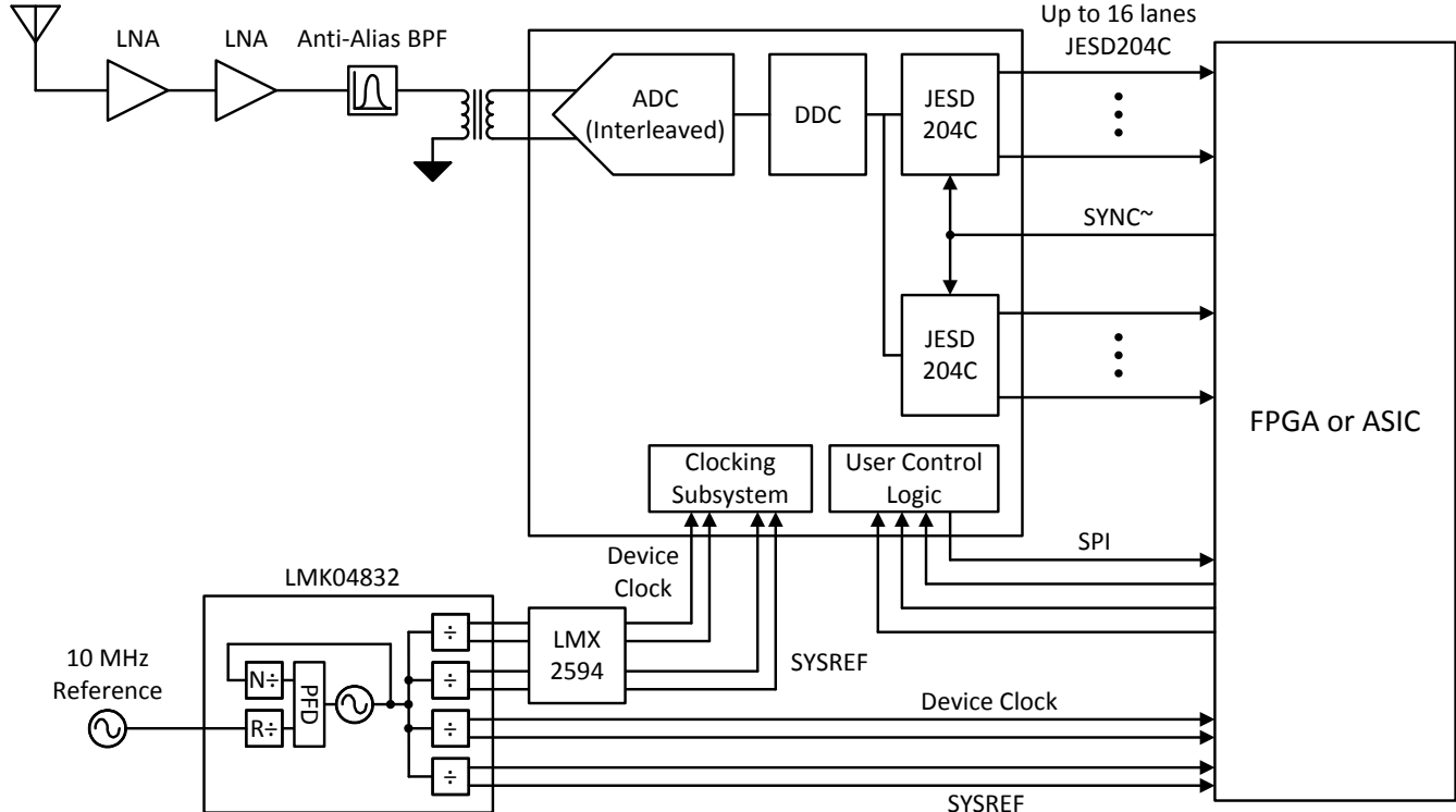
図 8-1. 広帯域 RF サンプリングの標準的な構成
