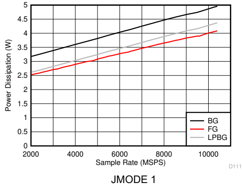
図 6-141. DES モード : 消費電力とサンプル レートとの関係
