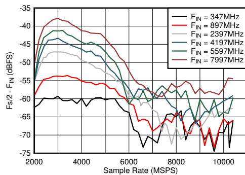
図 6-41. DES モード : F_s/2 - F_{IN} とサンプル レートおよび入力周波数との関係
