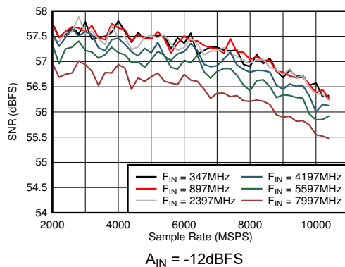
図 6-31. DES モード: SNR とサンプル レートおよび入力周波数との関係
