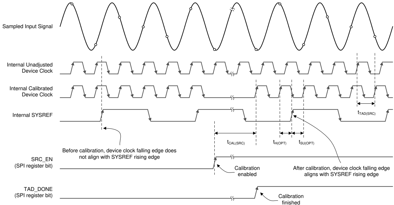
図 7-3. SYSREF 較正のタイミング図
