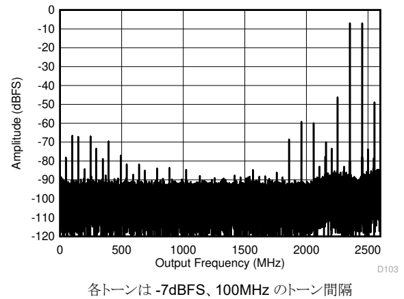
図 6-28. デュアルチャネルモード：2 トーン FFT (7997MHz で)
