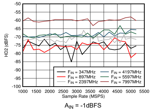
図 6-50. デュアル チャネル モード: HD2 とサンプル レートおよび入力周波数との関係
