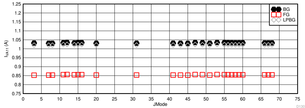
図 6-115. デュアル チャネル モード : I_{VA19} と JMODE (5.2GSPS) との関係
