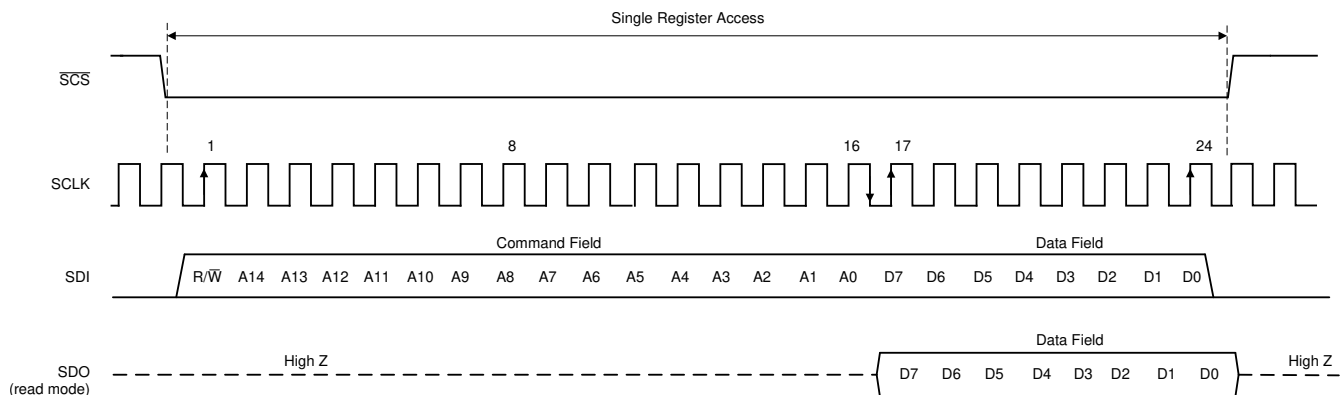
図 7-27. シリアル インターフェイス プロトコル : シングル読み取り / 書き込み
