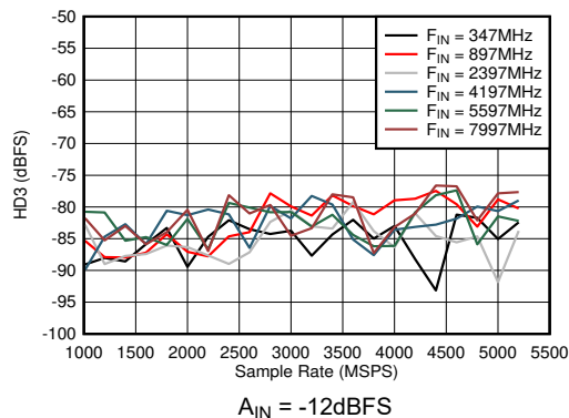
図 6-55. デュアル チャネル モード : HD3 とサンプル レートおよび入力周波数との関係
