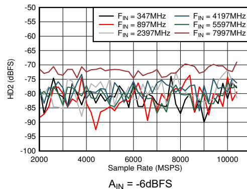
図 6-36. DES モード: HD2 とサンプル レートおよび入力周波数との関係
