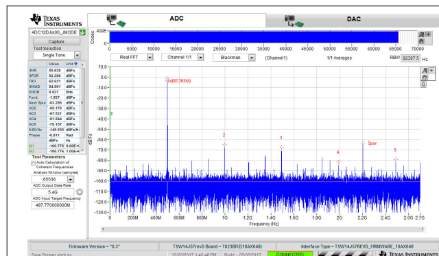
図 8-2. 497.77MHz 入力信号用 FFT、5.4GSPS、JMODE0
