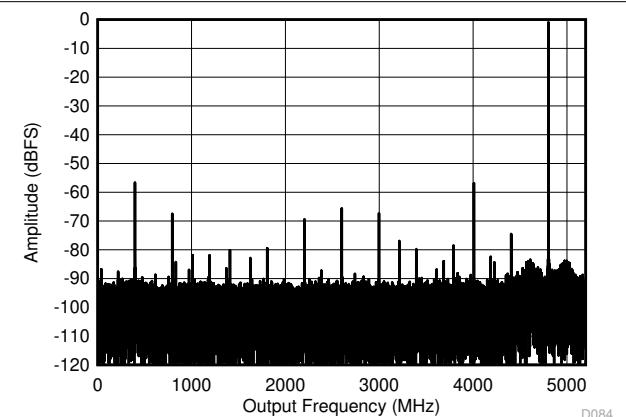
図 6-9. DES モード : 5597MHz でのシングル トーン FFT
