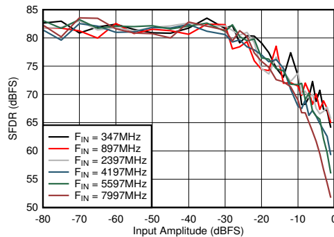
図 6-73. デュアル チャネル モード : SFDR と入力振幅および周波数との関係
