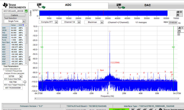
図 8-4. 497.77MHz 入力信号用 FFT、2.7GSPS、16 倍デシメーション、 f_{NCO} = 500\text{MHz} 、JMODE16
