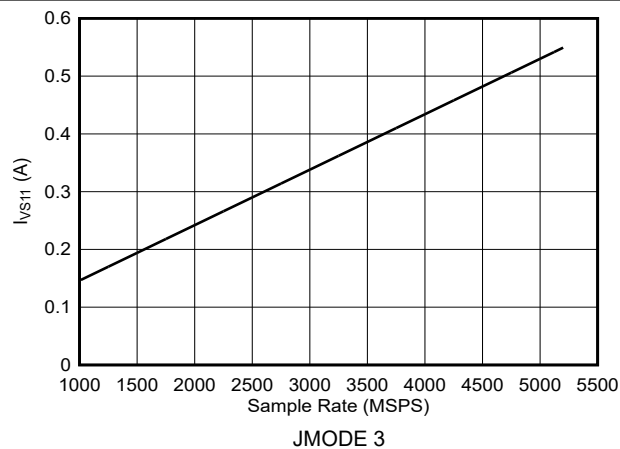
図 6-149. デュアル チャネル モード: I_{VS11} とサンプル レートとの関係 (ADC12DJ5210RF)
