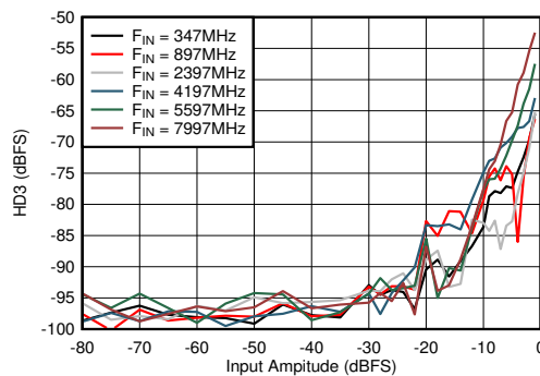
図 6-63. DES モード : HD3 と入力振幅および周波数との関係
