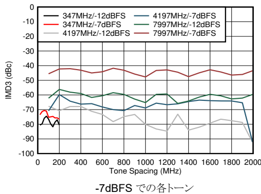
図 6-101. DES モード : IMD3 とトーン間隔との関係
