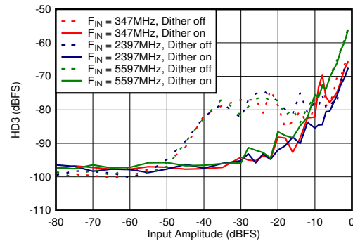
図 6-78. デュアル チャネル モード : HD3 と入力振幅およびディザとの関係
