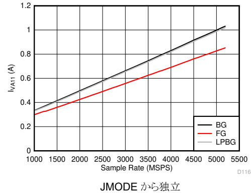
図 6-146. デュアル チャネル モード : I_{VA11} とサンプル レートとの関係
