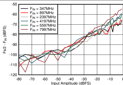
図 6-65. DES モード : F_s/2 - F_{\text{IN}} と入力振幅および周波数との関係
