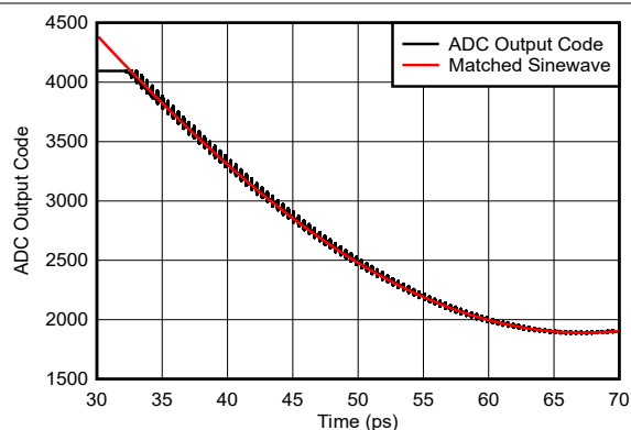
図 6-171. 正弦波オーバードライブ回復
