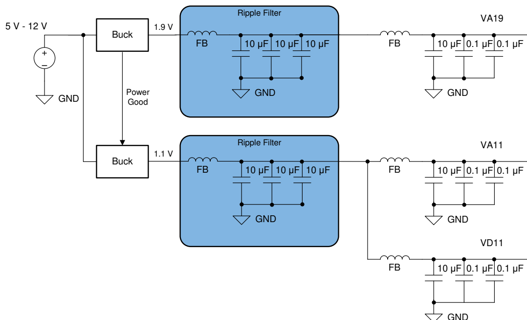
図 8-13. LDO リニア レギュレータのアプローチ例 (ADC12DJ5200RF)
