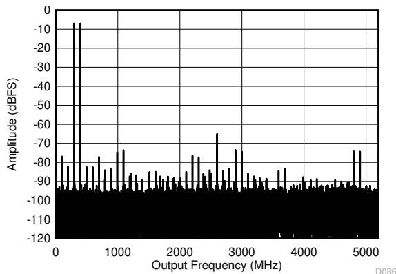
図 6-11. DES モード : 2 トーン FFT (347MHz で)
