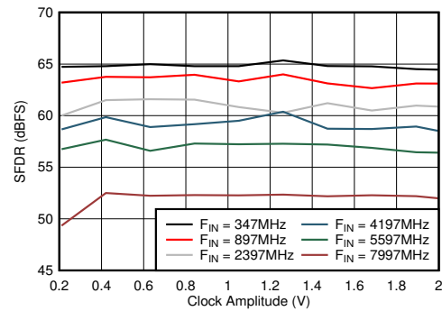
図 6-82. DES モード : SFDR とクロック振幅との関係
