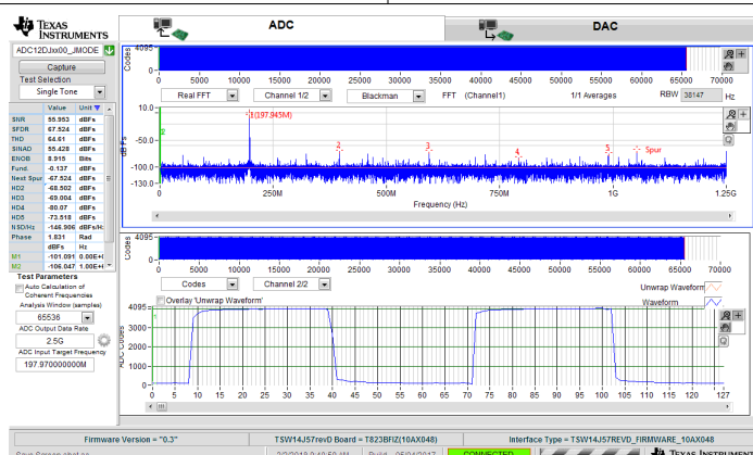
図 8-12. 5GSPS シングル チャネル オシロスコープにおける 200MHz、正弦波 (チャネル A) 周波数ドメイン (FFT) および 40MHz、方形波 (チャネル B) 時間ドメイン
