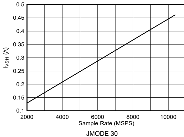
図 6-137. DES モード : I_{VS11} とサンプル レートとの関係 (ADC12DJ5210RF)
