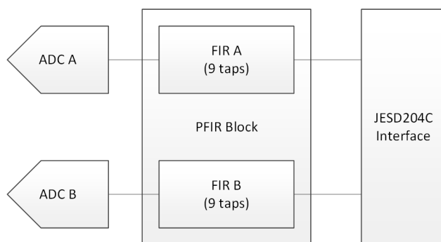
図 7-4. デュアル チャネル イコライゼーション PFIR のブロック図
