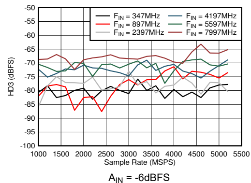
図 6-54. デュアル チャネル モード : HD3 とサンプル レートおよび入力周波数との関係
