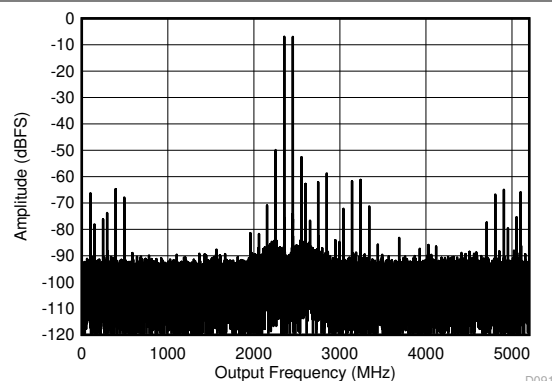
図 6-16. DES モード : 2 トーン FFT (7997MHz で)
