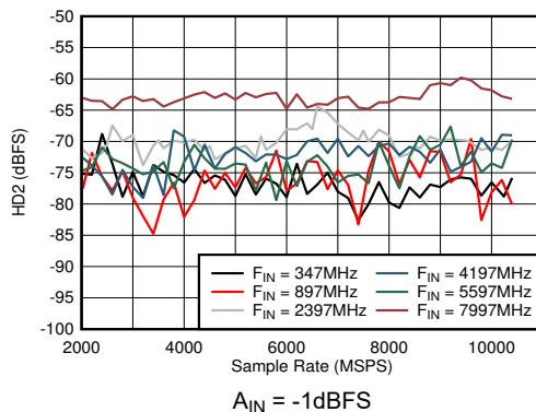
図 6-35. DES モード: HD2 とサンプル レートおよび入力周波数との関係
