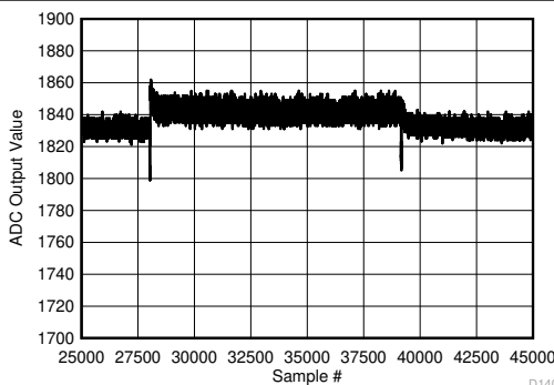
図 6-167. バックグラウンド キャリブレーション コアの遷移 (DC 信号 - 拡大)
