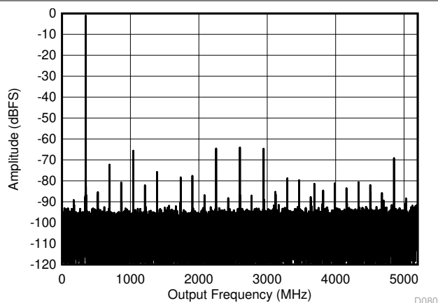
図 6-5. DES モード : 347MHz でのシングル トーン FFT
