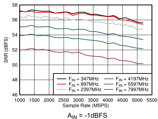
図 6-44. デュアル チャネル モード : SNR とサンプル レートおよび入力周波数との関係
