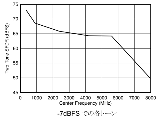
図 6-102. DES モード : 2 トーン SFDR と入力周波数との関係
