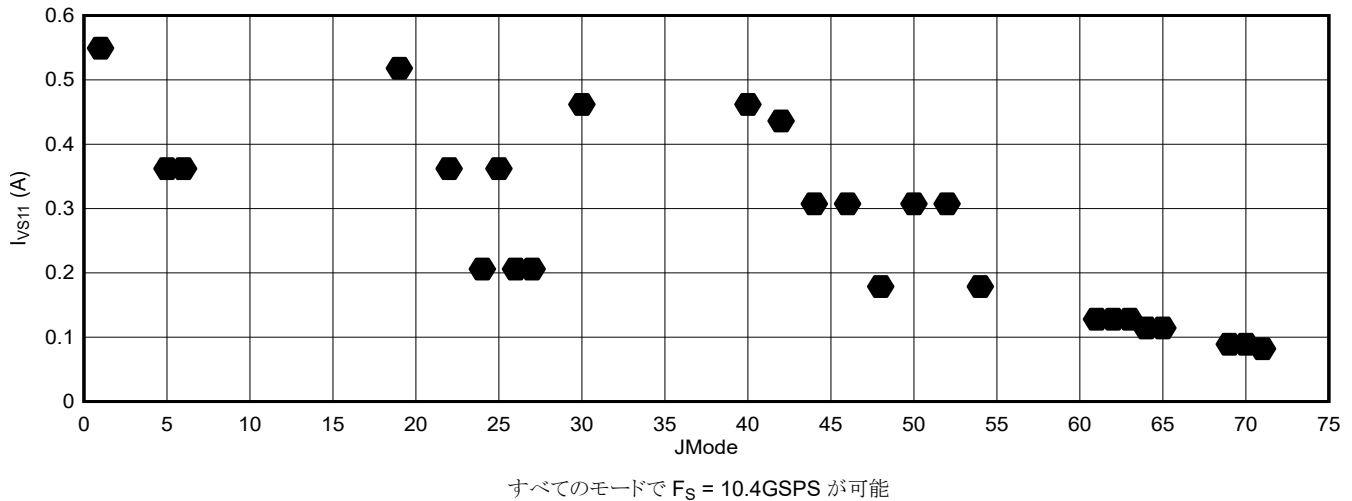
図 6-113. DES モード : I_{VS11} と JMODE (10.4GSPS) との関係 (ADC12DJ5210RF)
