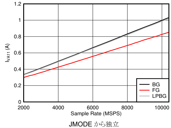
図 6-128. DES モード : I_{VA11} とサンプル レートとの関係
