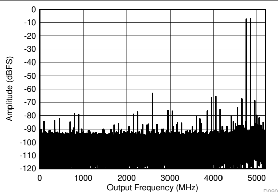
図 6-15. DES モード : 2 トーン FFT (5597MHz で)
