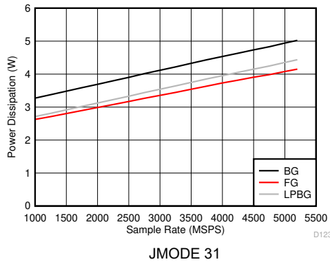
図 6-161. デュアルチャネル モード：消費電力とサンプル レートとの関係
