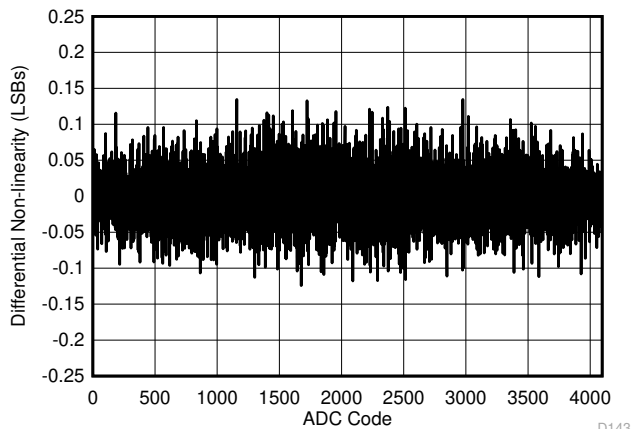
図 6-3. DNL と ADC コードとの関係
