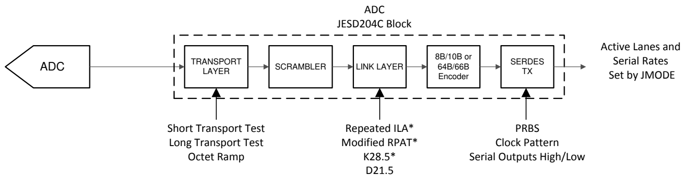
図 7-25. テスト・モードの挿入ポイント
