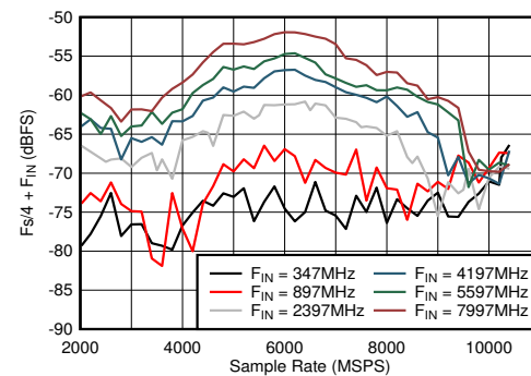
図 6-42. DES モード : F_s/4 + F_{IN} とサンプル レートおよび入力周波数との関係
