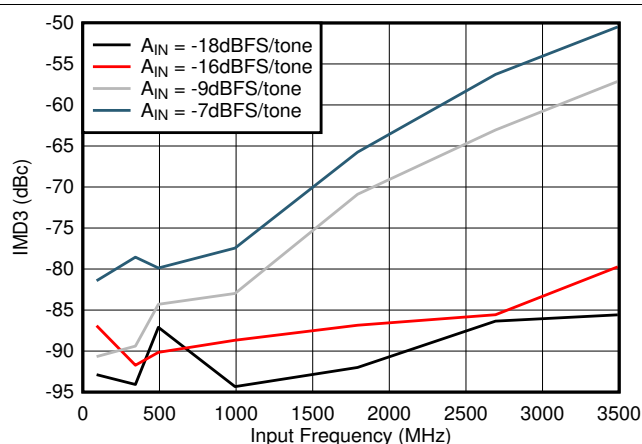
図 5-72. IMD3 vs Input Frequency
