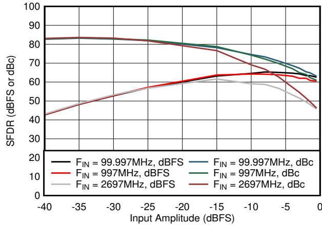
図 5-33. SFDR vs Input Amplitude
