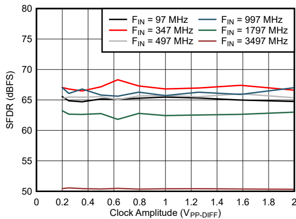
図 5-41. SFDR vs Clock Amplitude
