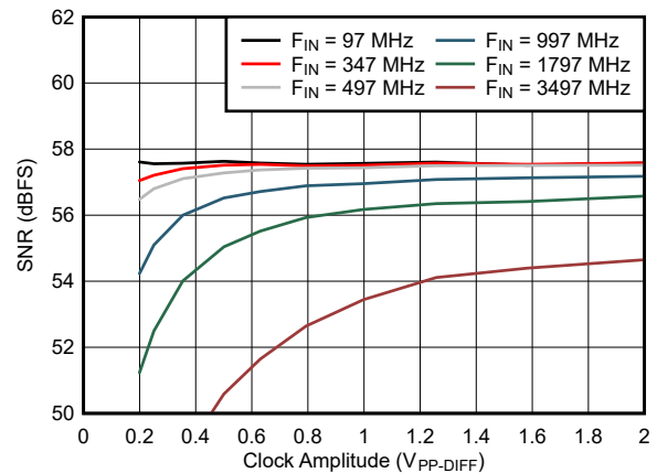
図 5-40. SNR vs Clock Amplitude
