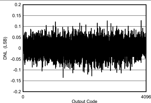
図 5-1. DNL vs Code
