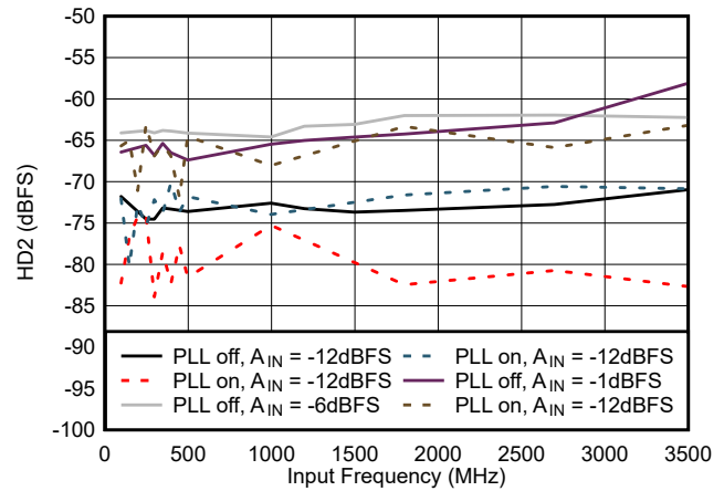
図 5-24. HD2 vs Input Frequency
