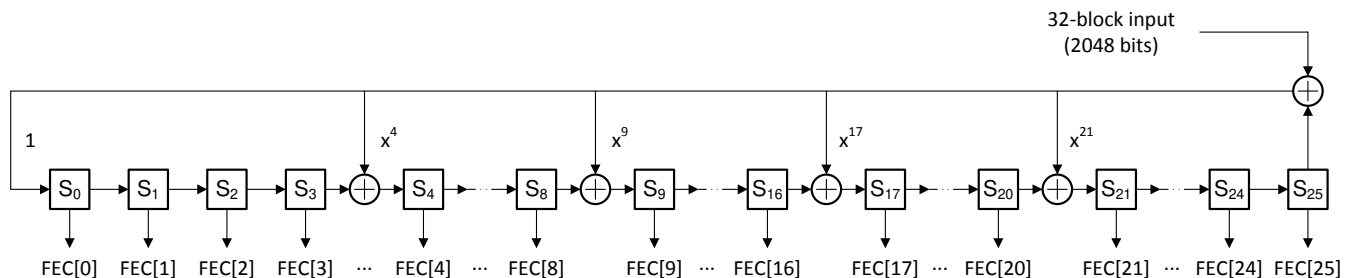
図 7-10. FEC Parity Bit Generator
