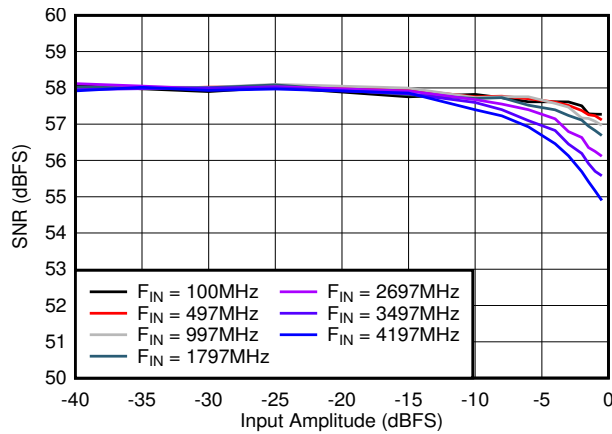
図 6-33. SNR vs A_{IN}
