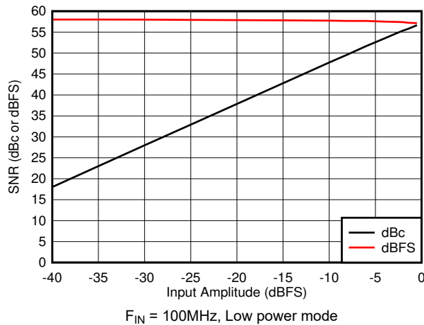
図 6-35. SNR vs A_{IN}
