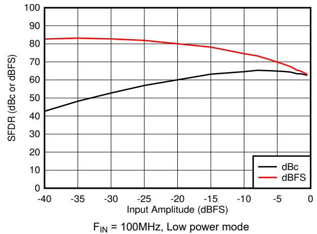
図 5-34. SFDR vs A_{IN}
