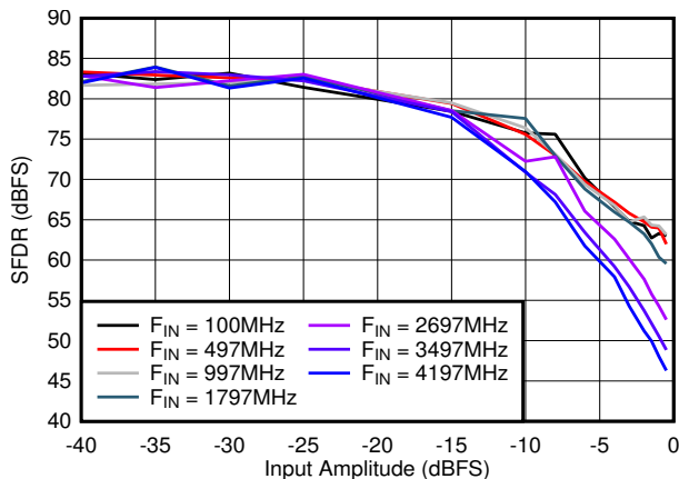
図 5-32. SFDR vs A_{IN}
