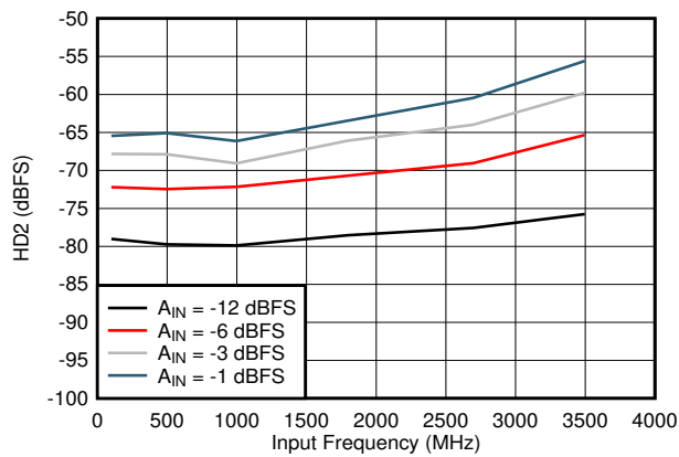
図 5-21. HD2 vs Input Frequency
