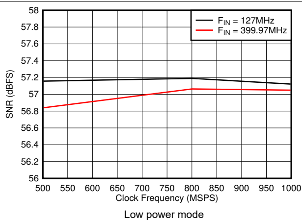
図 5-28. SNR vs Sample Rate
