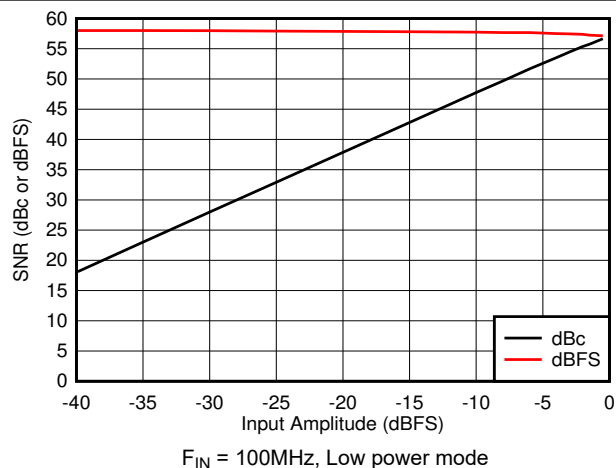
図 5-35. SNR vs A_{IN}
