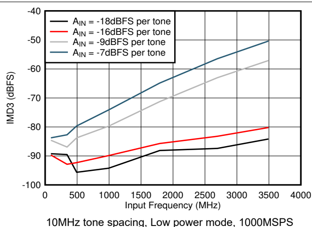
図 5-76. IMD3 vs F_{IN}
