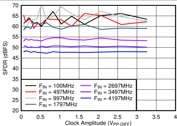
図 5-36. SFDR vs A_{CLK}
