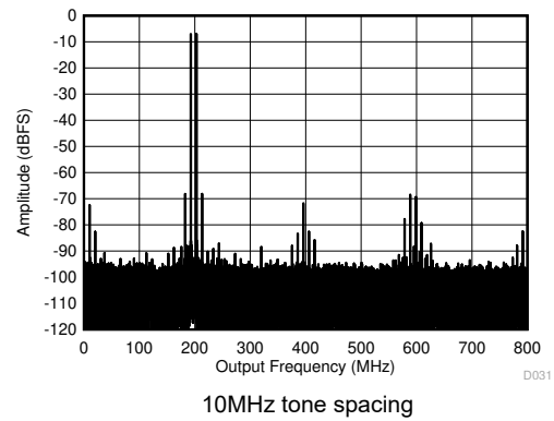
図 5-70. Two Tone FFT at 1798MHz
