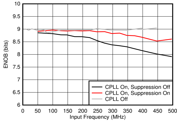
図 5-47. ENOB と F_{IN} および C-PLL モード
