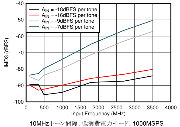
図 5-76. IMD3 と F_{IN} との関係
