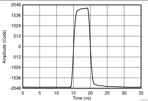
図 7-2. 32GSPS 等価測定でサブサンプリング手法を使用したパルス測定
