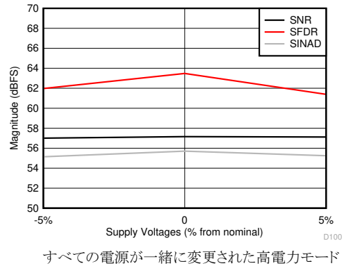
図 5-60. SNR、SFDR、SINAD と電源電圧との関係
