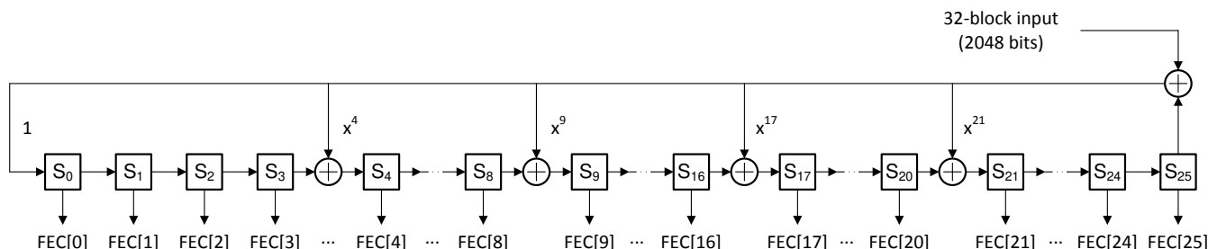
図 6-8. FEC パリティビットジェネレータ
