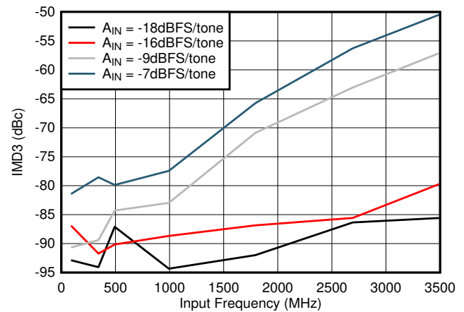
図 5-72. IMD3 vs Input Frequency
