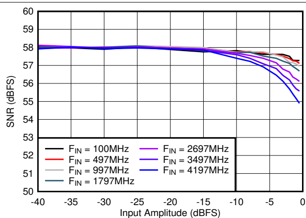
図 5-33. SNR vs A_{IN}
