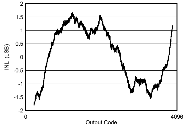
図 5-2. INL vs Code
