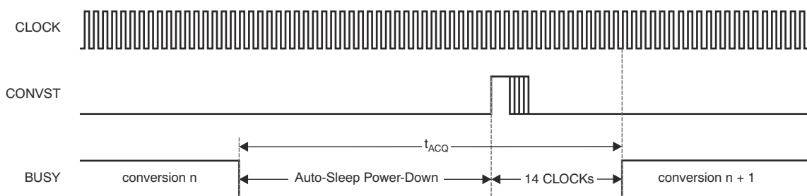
6-4. Actual Conversion Start In Auto-Sleep Mode
