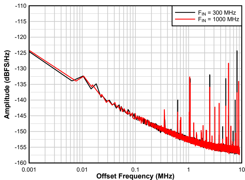
図 7-8. Amplitude Noise
