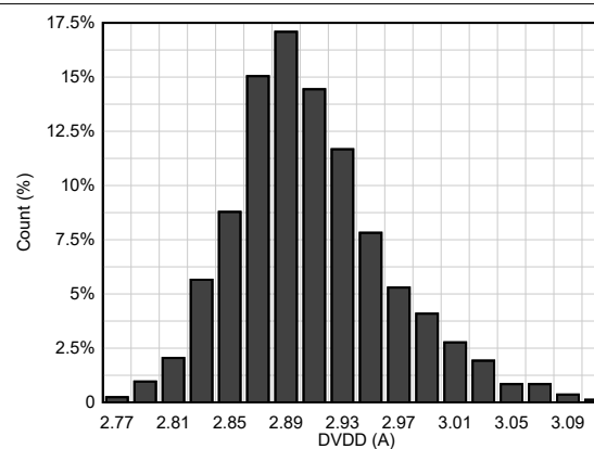
图 6-115. DVDD Distribution
