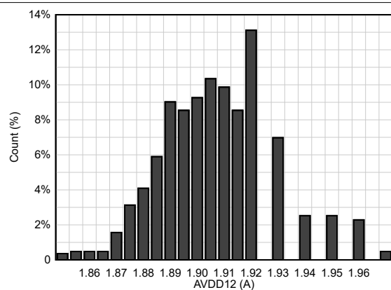
图 6-114. AVDD12 Distribution
