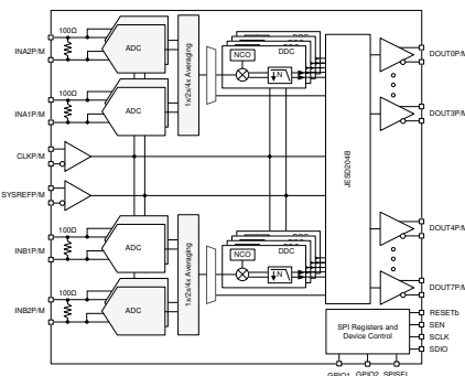
ブロック図
