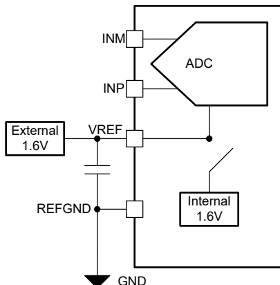
図 7-9. 外部リファレンス モード
