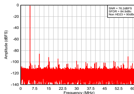
シングル トーン スペクトル、 F_s = 125\text{MSPS} 、 F_{in} = 5\text{MHz}
