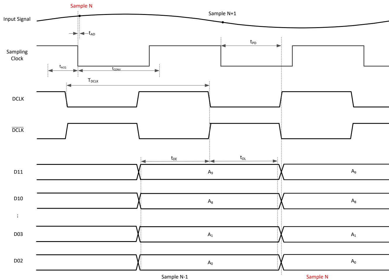
図 5-2. Timing Diagram: 10-Bit SDR (Default: 10 Lanes)
