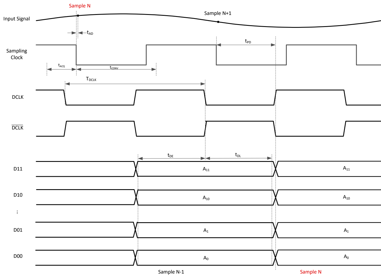
図 5-4. Timing Diagram: 12-Bit SDR (Default: 10 Lanes)
