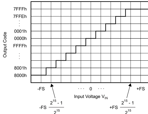
図 35. Code Transition Diagram
