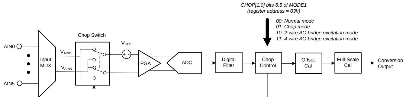
✎ 59. ADC Chop Mode
