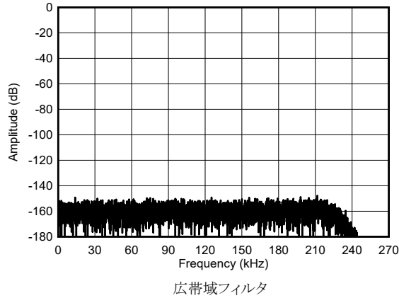
図 5-7. 最高速度モード、短絡入力 FFT
