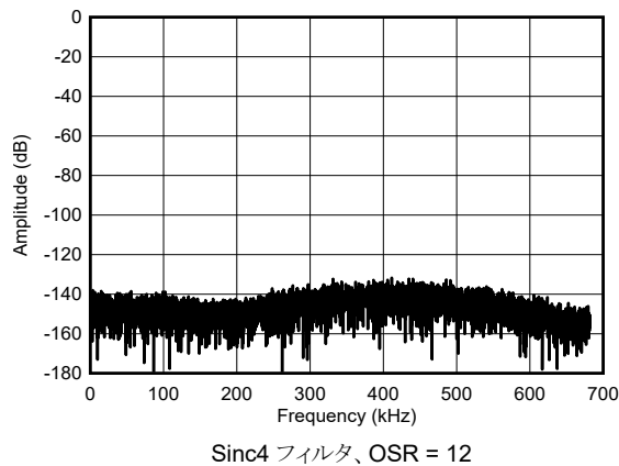
図 5-11. 最高速度モード、短絡入力 FFT
