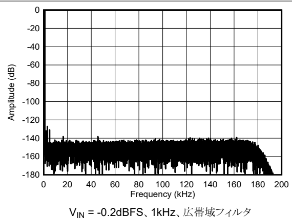
図 5-18. 高速度モード、フルスケール FFT
