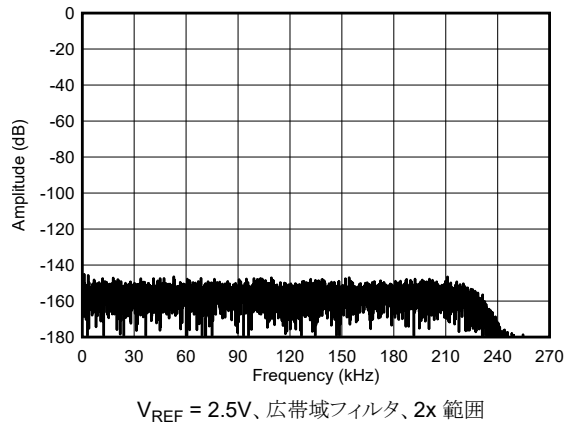
図 5-9. 最高速度モード、短絡入力 FFT
