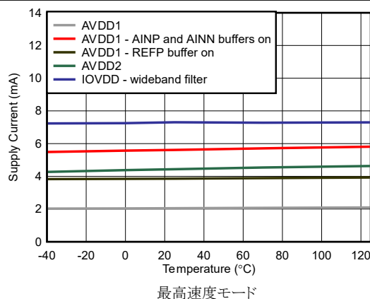
図 5-82. 電源電流と温度との関係
