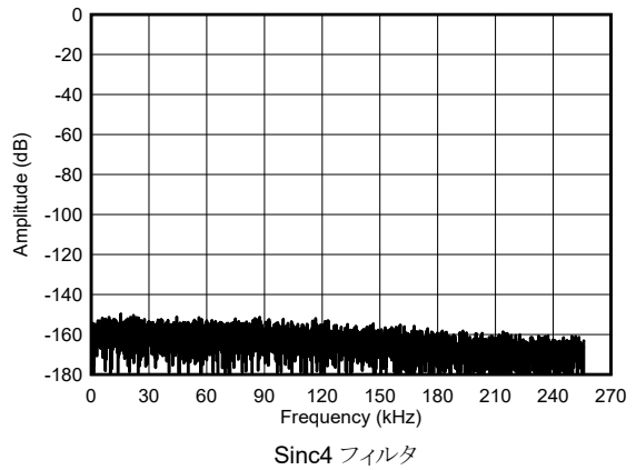
図 5-10. 最高速度モード、短絡入力 FFT
