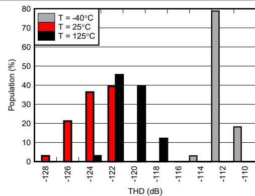
図 5-58. THD の分布
