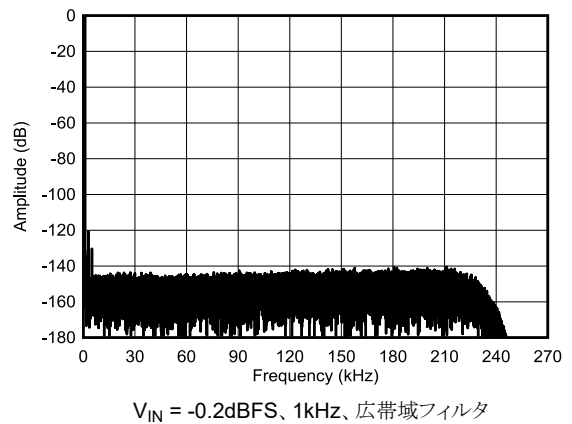
図 5-12. 最高速度モード、フルスケール FFT
