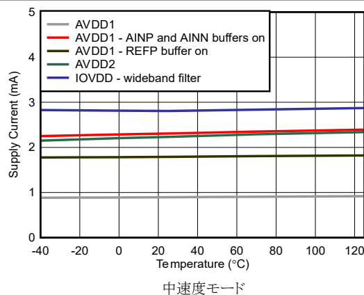
図 5-84. 電源電流と温度との関係
