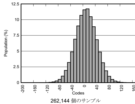
図 5-34. 低速度モードのコード分布
