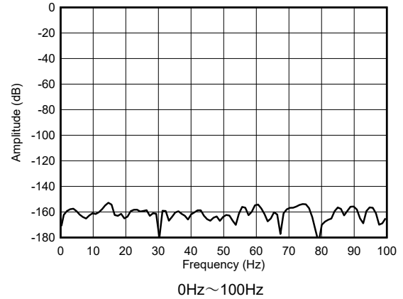
図 5-8. 最高速度モード、短絡入力 FFT
