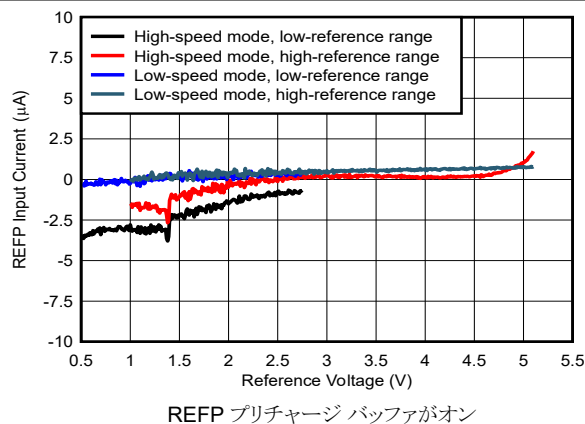
図 5-78. REFP 入力電流とリファレンス電圧との関係
