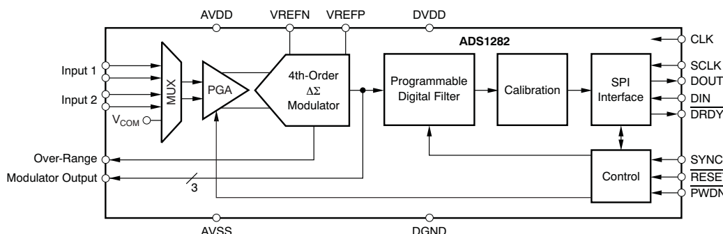
概略回路図
