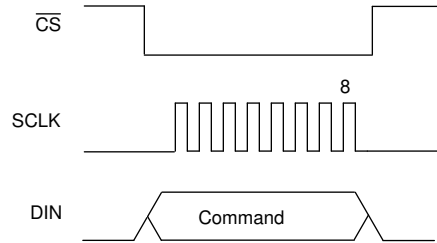
図 7-23. シングル バイトのコマンド形式
