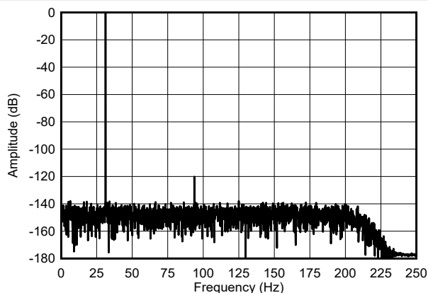
図 5-23. 中電力モードの FFT スペクトル
