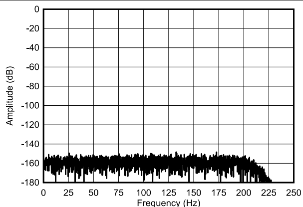
図 5-28. 低電力モードの FFT スペクトル
