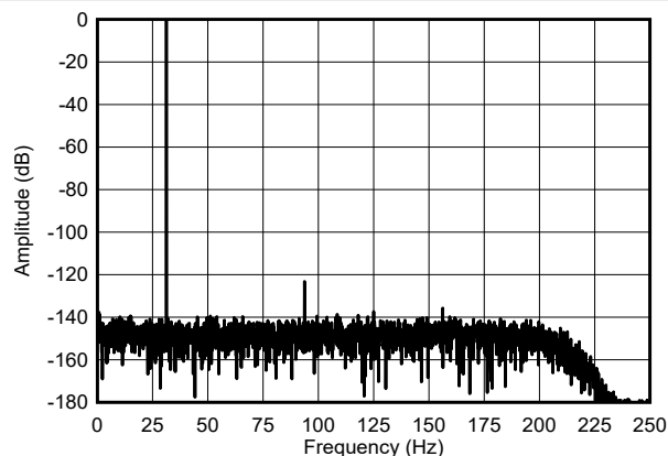
図 5-31. 低電力モードの FFT スペクトル
