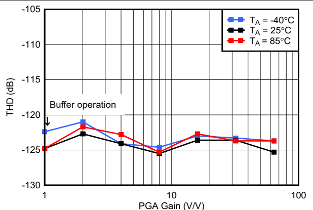
図 5-48. 低電力モード THD と PGA ゲインとの関係
