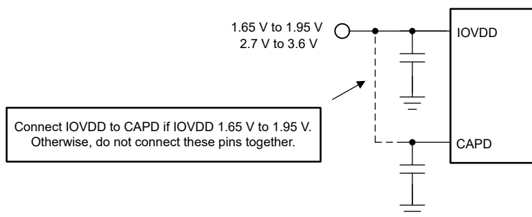
図 7-9. IOVDD 電源の接続
