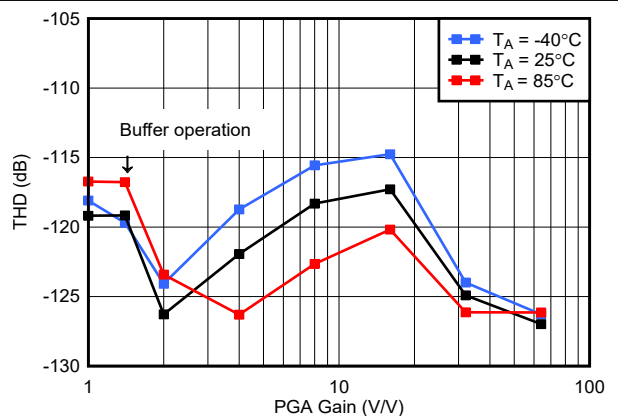
図 5-47. 中電力モード THD と PGA ゲインとの関係
