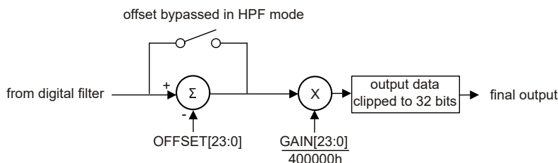
図 7-20. 校正のブロック図
