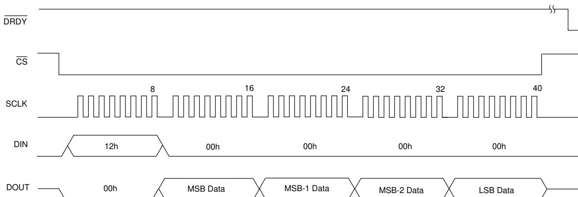
図 7-25. コマンドにより変換データを読み取り
