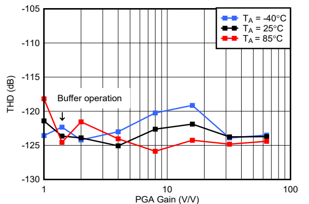
図 5-49. ハイパワー モード THD と PGA ゲインとの関係
