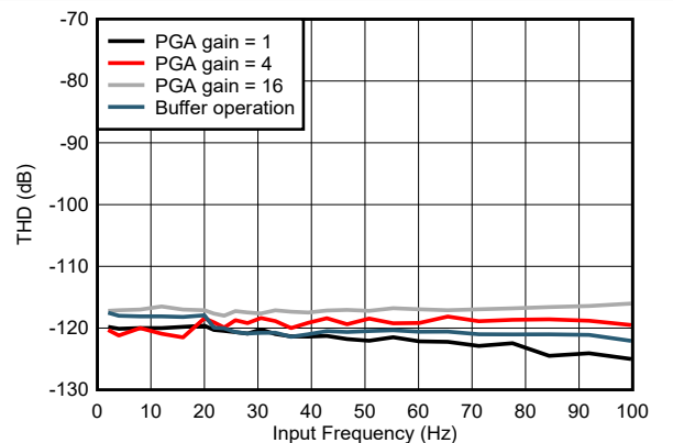
図 5-50. 中電力モード THD と PGA ゲインとの関係
