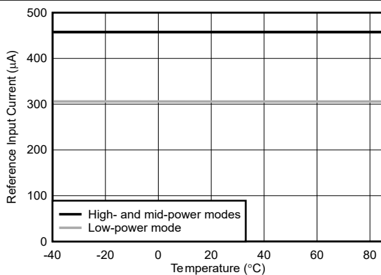
図 5-57. リファレンス入力電流と温度との関係
