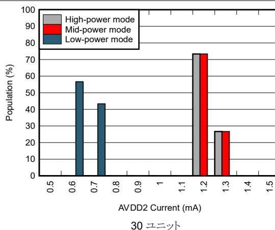
図 5-64. AVDD2 電流の分布
