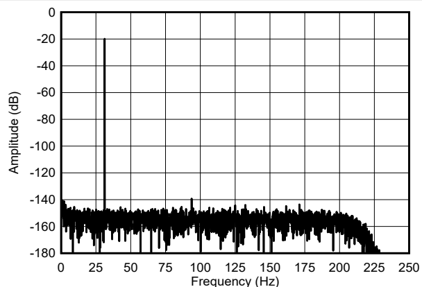
図 5-32. 低電力モードの FFT スペクトル
