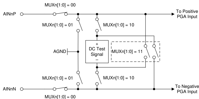
FIG 8-2. Input Multiplexer
