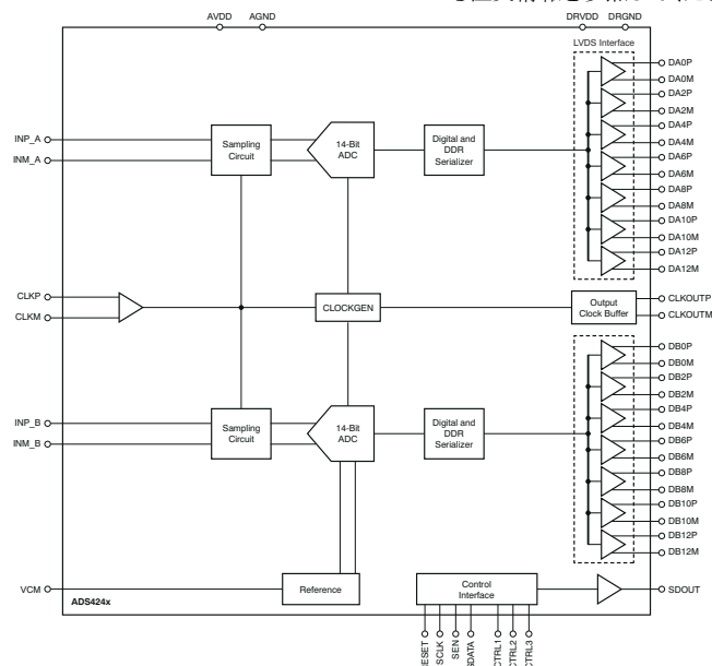
ADS4222、25、26、42、45、46 ブロック図
