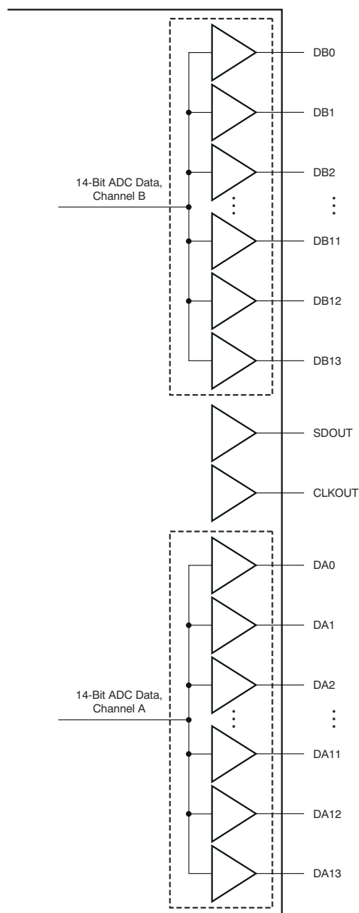
图 8-24. CMOS Outputs
