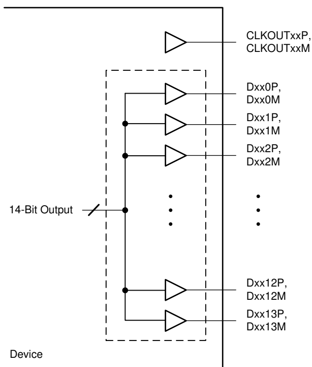
8-3. DDR LVDS Interface
