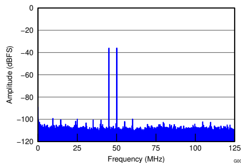
FIG 6-7. FFT for 230-MHz Input Signal
