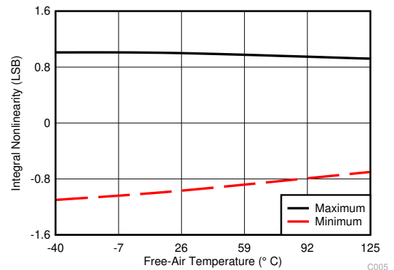
図 6-4. Typical INL
