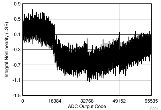
図 6-4. Typical INL
