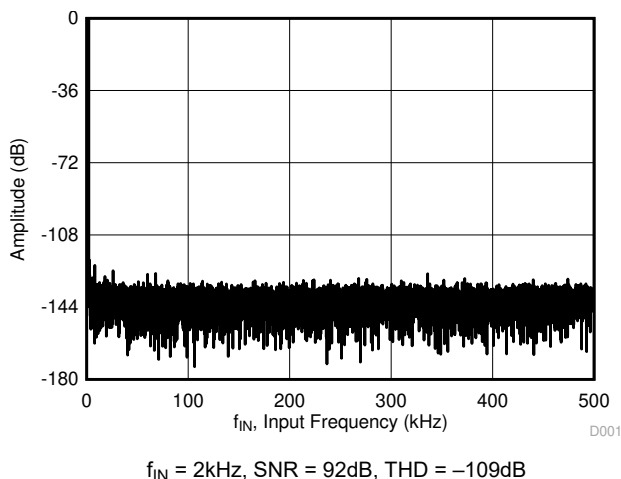
図 8-5. FFT Plot: ADS8168
