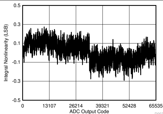
図 5-6. Typical INL
